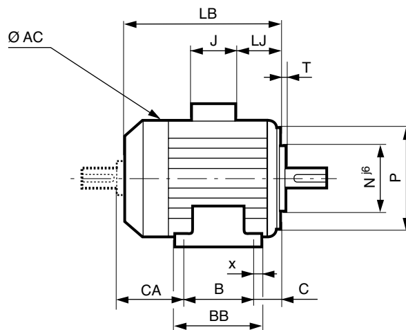
Dimensions principales
