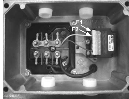
Klemmen F1 en F2 van de optie ESFR VMA 31/32
