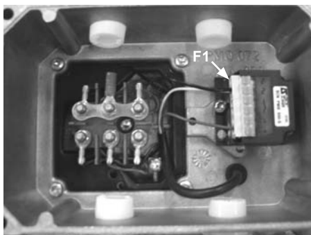
Klem F1 van de optie SO VMA 31/32
