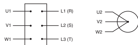
Fig. 11 - Raccordement tableau
