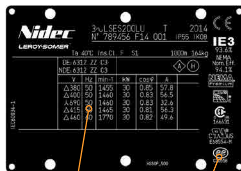
Identificatieplaatje IMfinity® IE3
