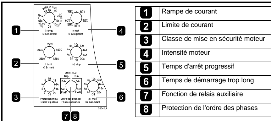
Figure 5-1 Commutateurs de réglage
