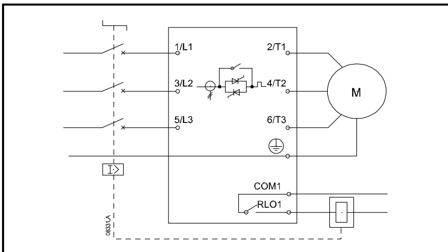
Figure 4-5 Démarreur progressif avec disjoncteur magnéto-thermique et contacteur principal
