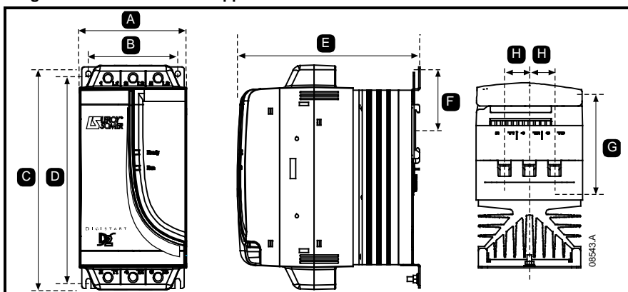
Figure 3-1 Dimensions de l'appareil
