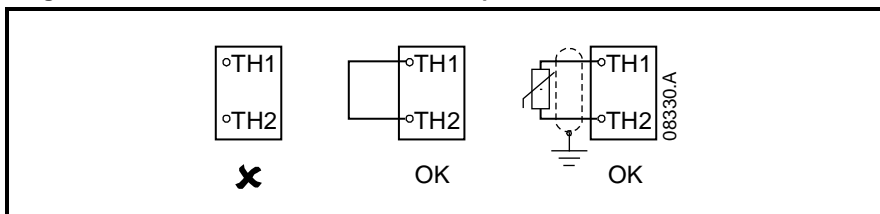
Figure 4-3 Raccordement des sondes thermiques moteur
