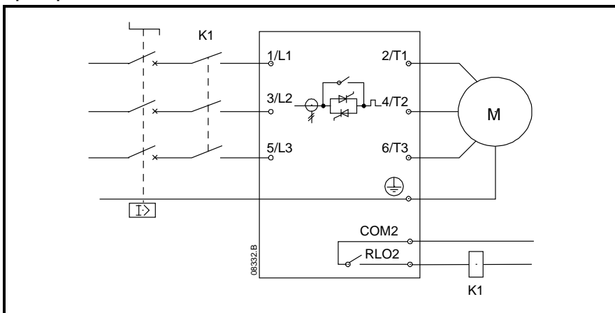
Figure 4-5 Démarreur progressif avec disjoncteur magnéto-thermique et contacteur principal
