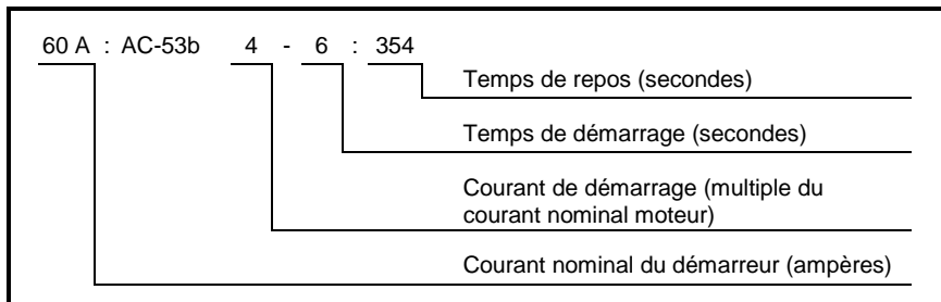
Figure 2-2 Code d'utilisation AC53b
