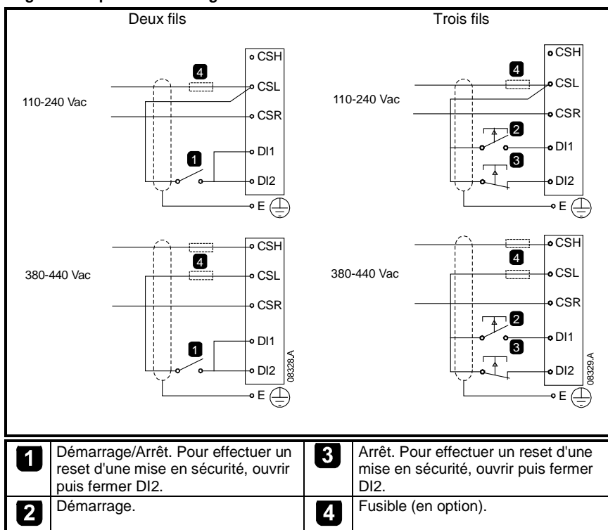
Figure 4-2 Options de câblage de commande
