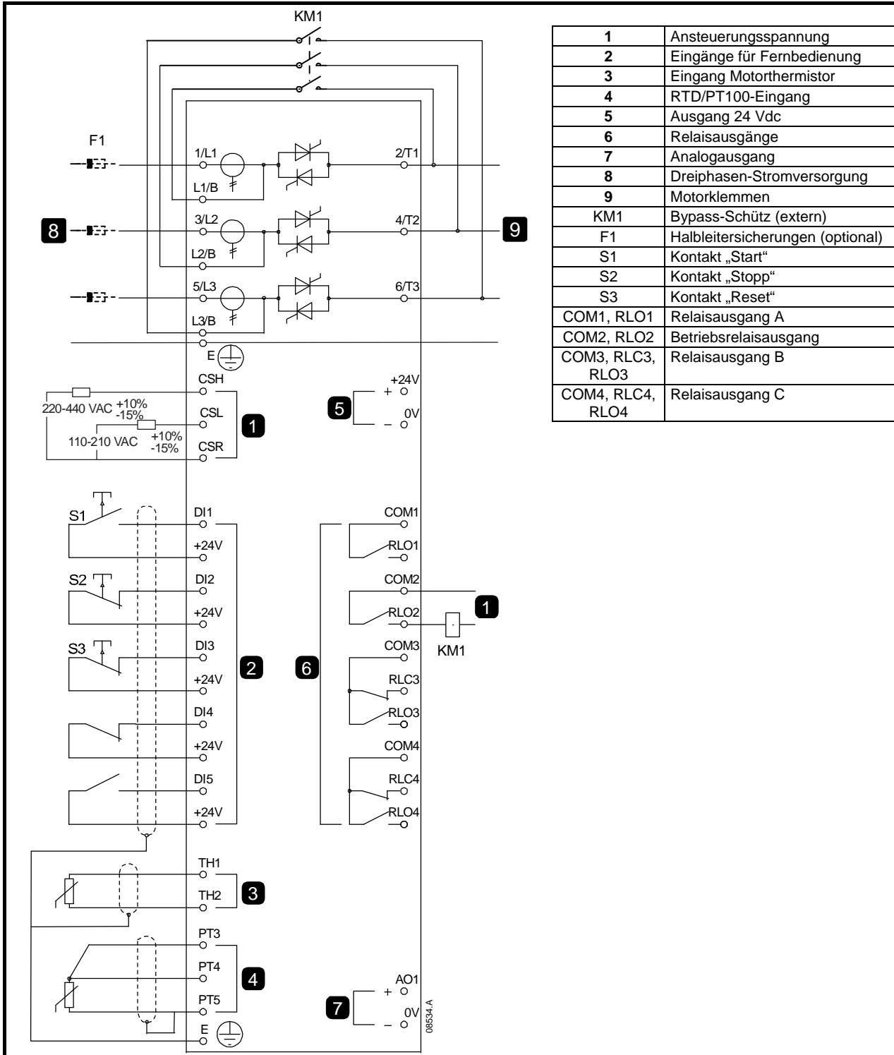
Abbildung 10-2 Installation mit Bypass-Schütz
