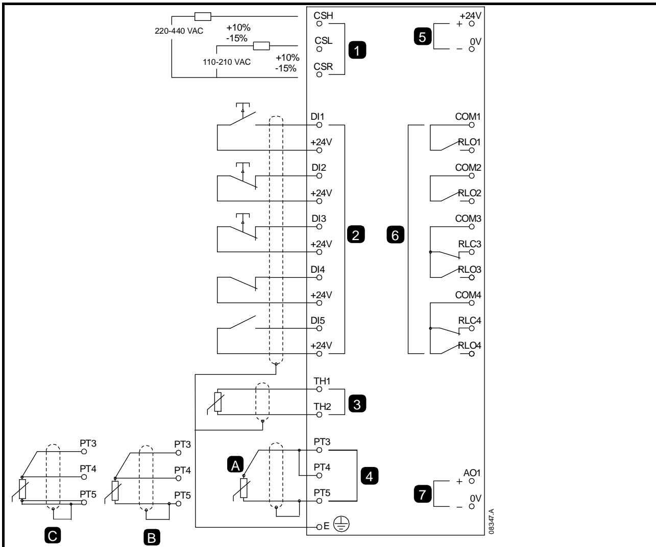
Abbildung 4-8 Digistart D3 - Elektroschaltbilder
