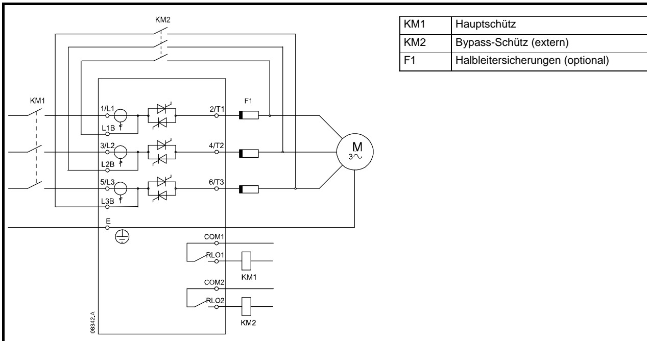
Abbildung 4-11 Hochspannungsanschlüsse – In-line-Installation, externer Bypass (D3-1x-0360-N bis D3-16-1600-N)
