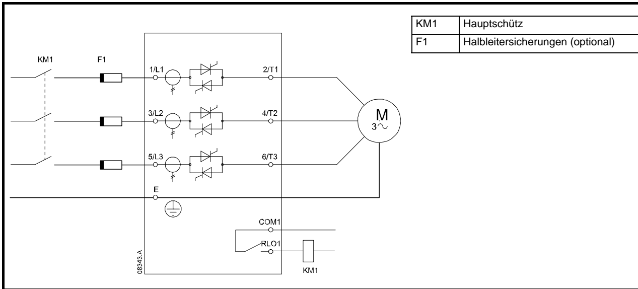
Abbildung 4-12 Hochspannungsanschlüsse - In-line-Installation, ohne Bypass
