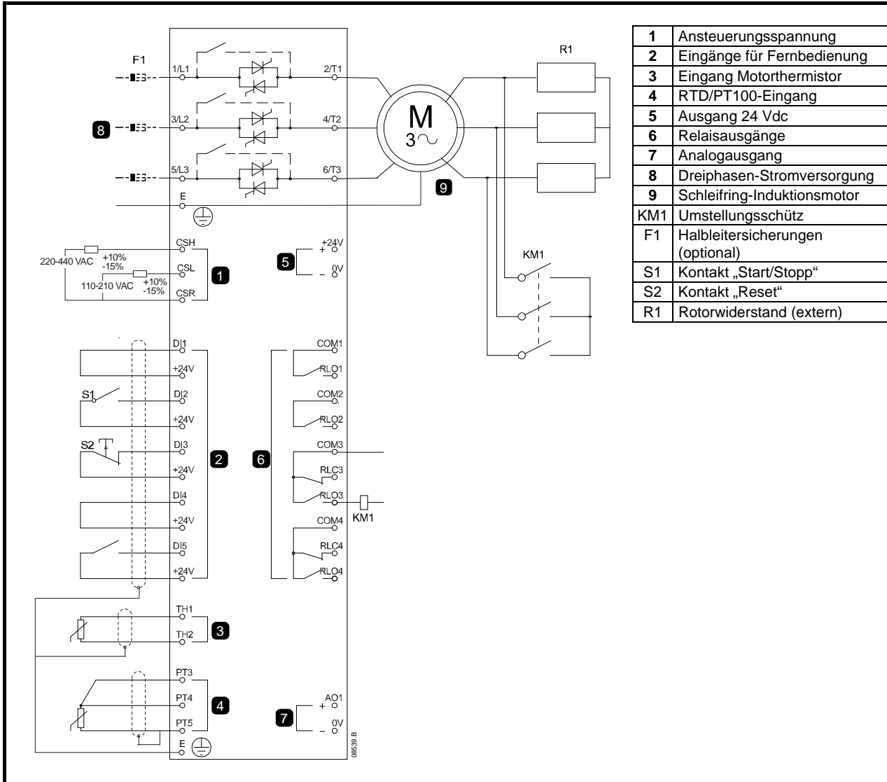
Abbildung 10-8 Schleifringmotor
