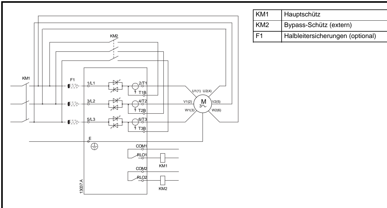
Abbildung 4-14 Hochspannungsanschlüsse – In-delta-Installation, externer Bypass (D3-1x-0255-N)
