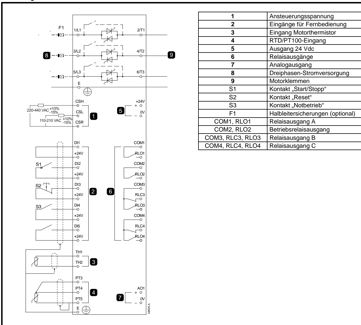
Abbildung 10-3 Notbetrieb
