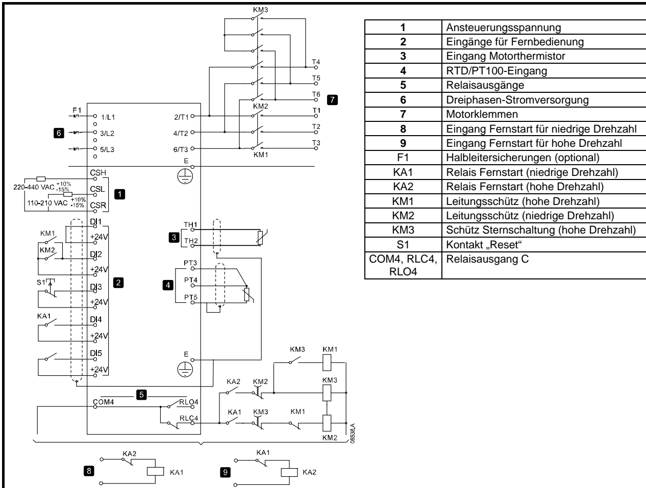
Abbildung 10-7 Motor mit zwei Drehzahlen
