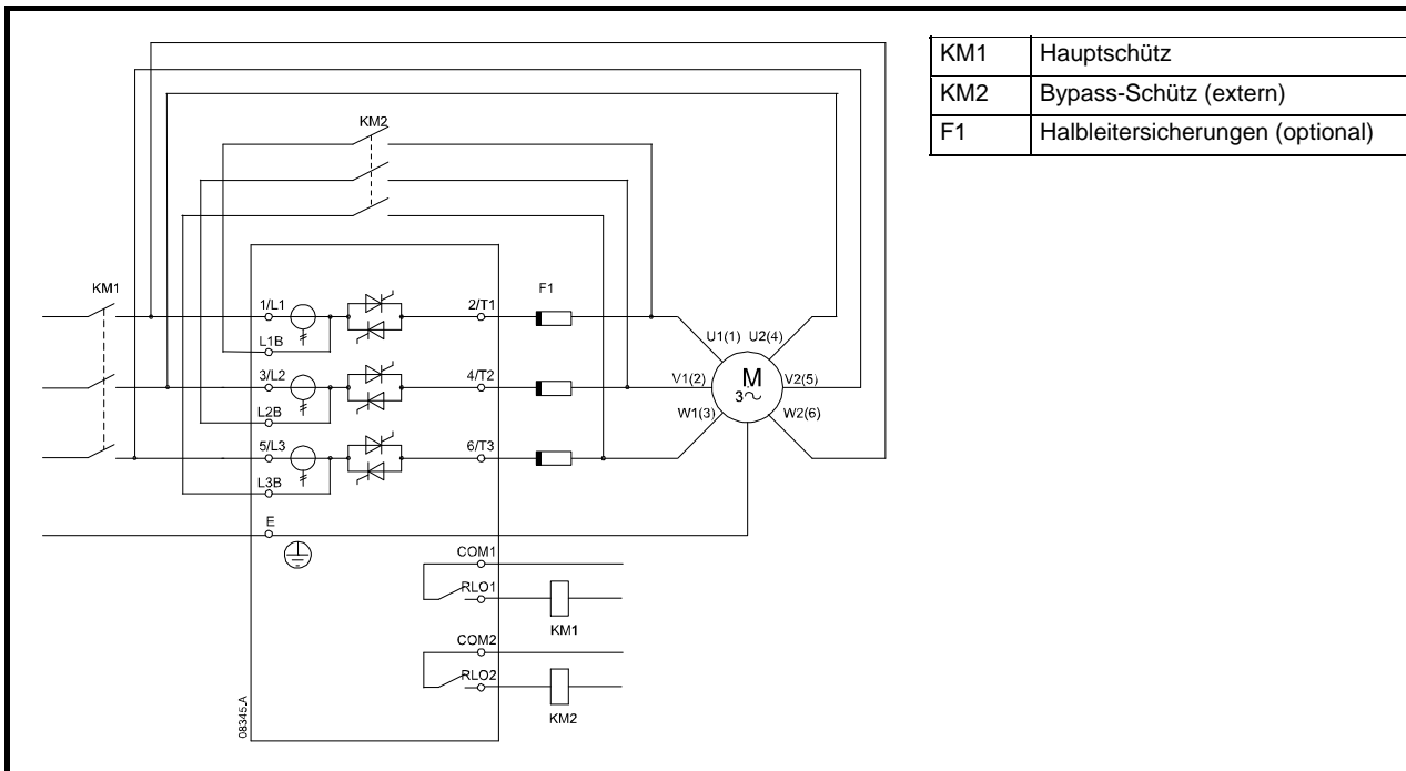
Abbildung 4-15 Hochspannungsanschlüsse – In-delta-Installation, externer Bypass (D3-1x-0360-N bis D3-16-1600-N)
