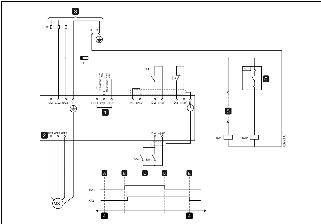
Abbildung 10-5 Gleichstrombremse mit externem Stoppsensor
