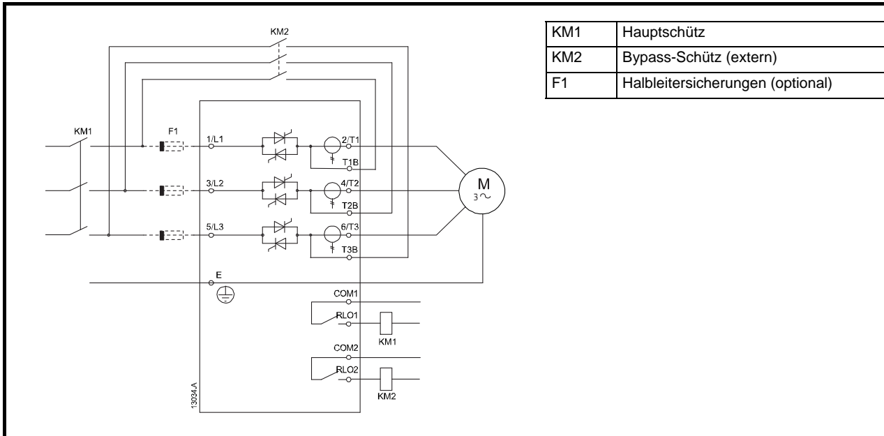
Abbildung 4-11 Hochspannungsanschlüsse – In-line-Installation, externer Bypass (D3-1x-0360-N bis D3-16-1600-N)
