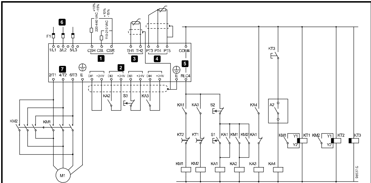
Abbildung 10-6 Soft-Bremsen
