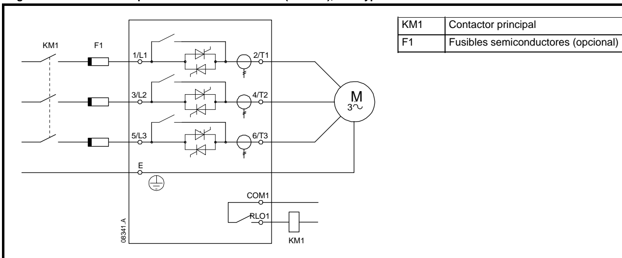
Figura 4-9 Conexiones de potencia - instalación directa (en línea), con bypass interno
