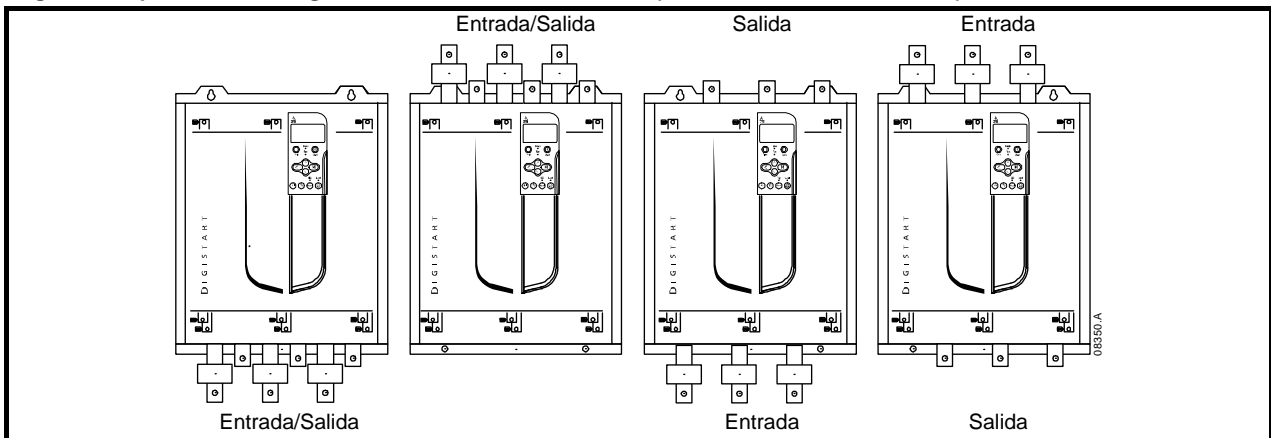
Figura 3-4 Opciones de configuración de las barras colectoras (D3-1x-0360-N a D3-16-1600-N)
