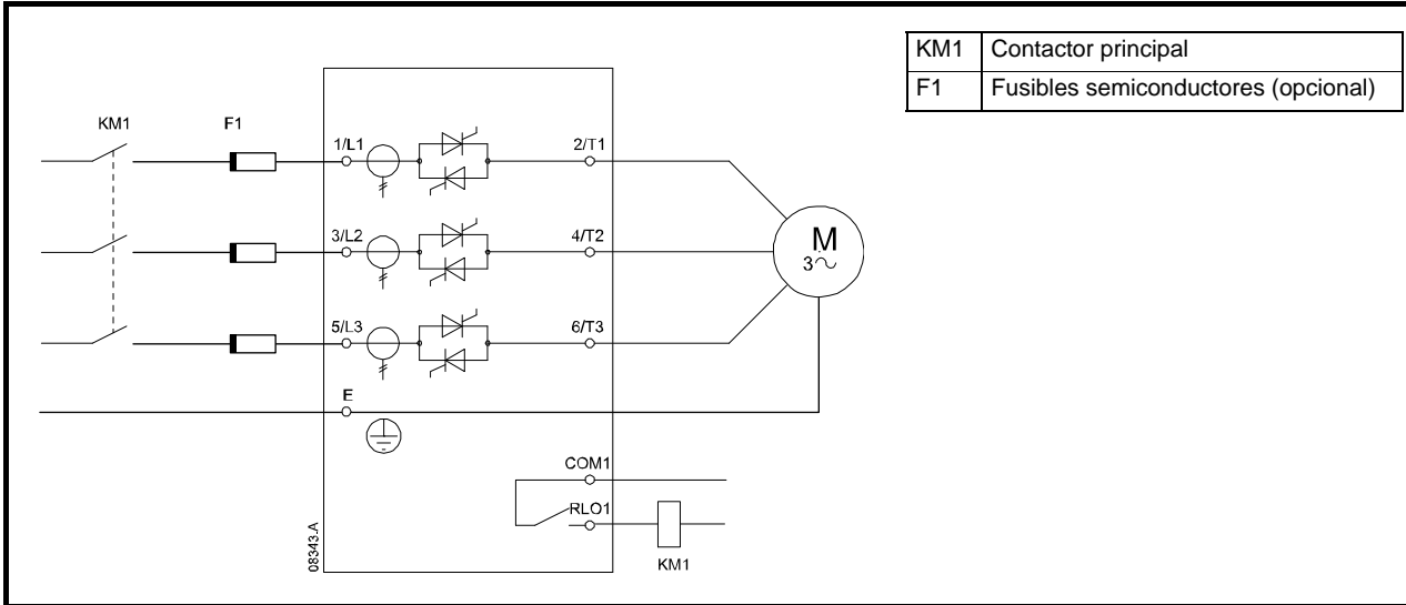
Figura 4-12 Conexiones de potencia - instalación directa (en línea), sin bypass
