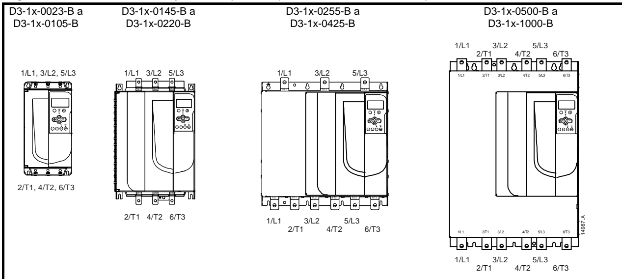
Figura 4-1 Terminales de entrada y salida de potencia (D3-1x-0023-B a D3-1x-1000-B)
