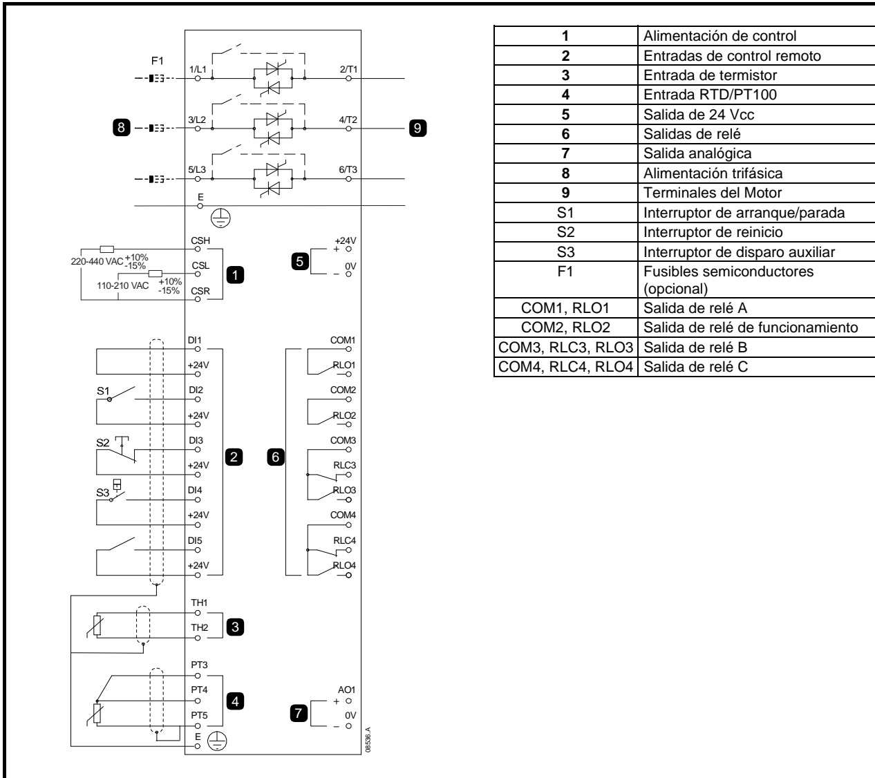
Figura 10-4 Circuito de disparo auxiliar
