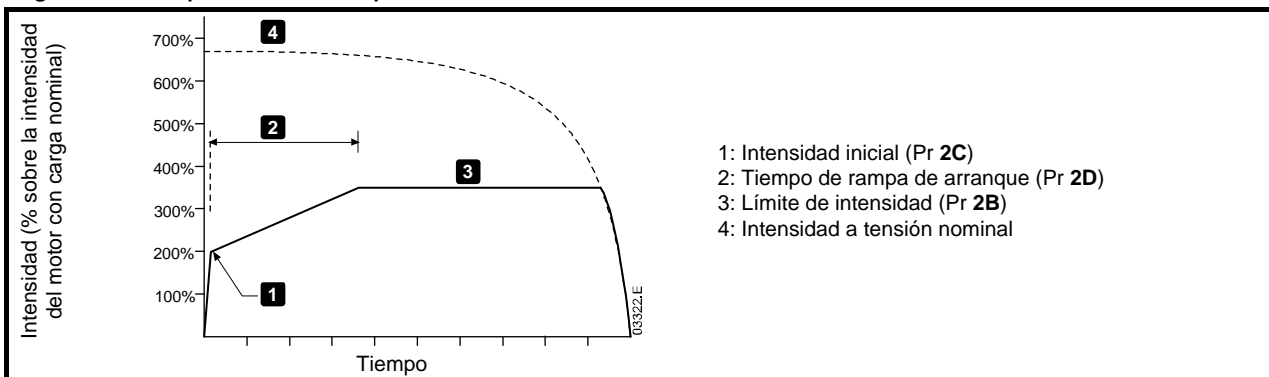
Figura 7-2 Arranque suave con rampa de intensidad
