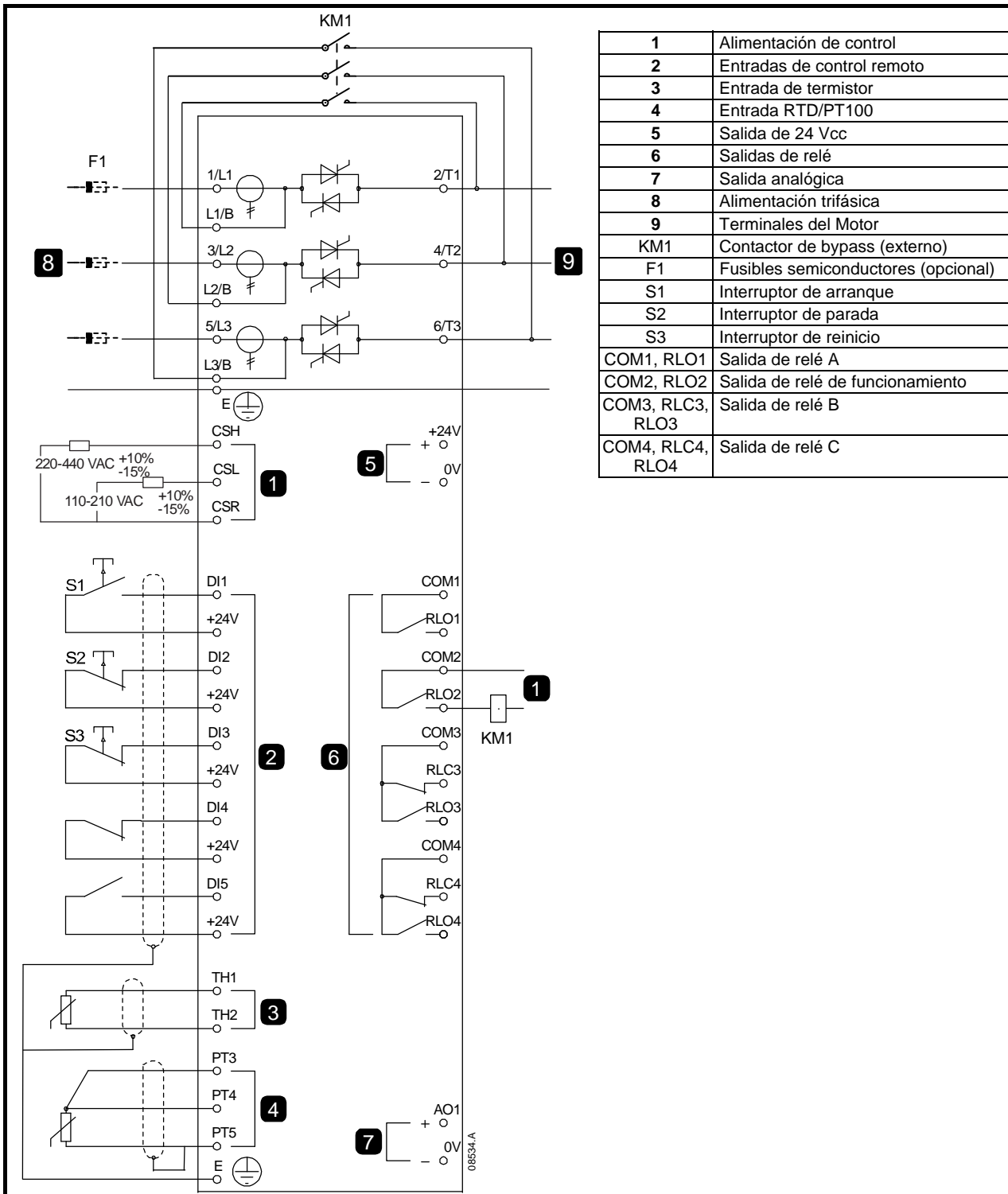
Figura 10-2 Instalación con interruptor de bypass
