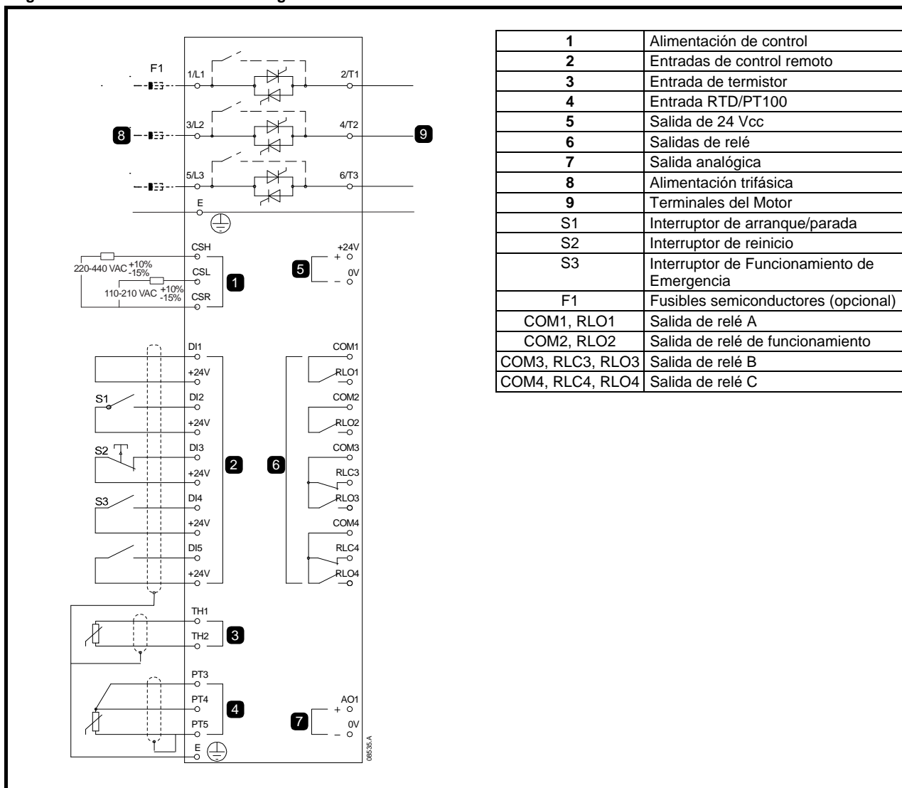
Figura 10-3 Funcionamiento de emergencia
