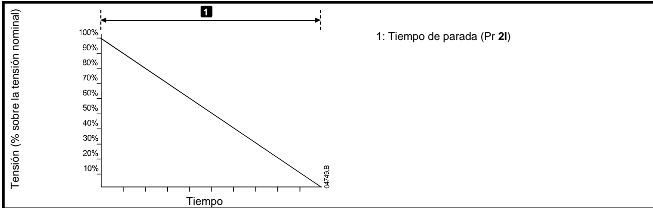
Figura 7-5 Parada suave TVR
