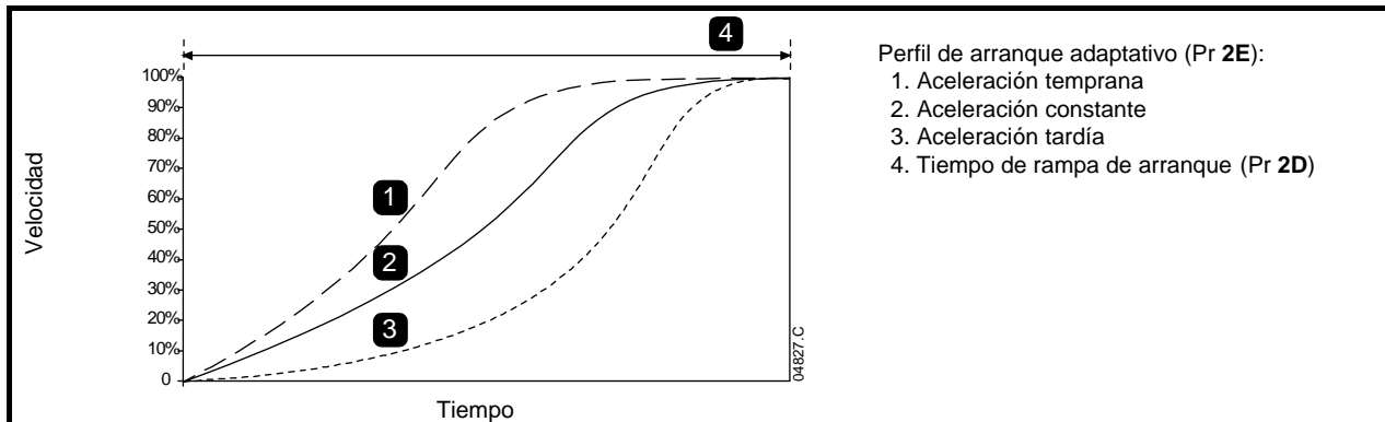
Figura 7-3 Arranque suave con Control Adaptativo
