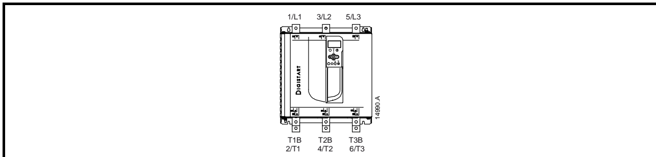
Figura 4-2 Terminales de potencia de entrada y salida (D3-1x-0255-N)
