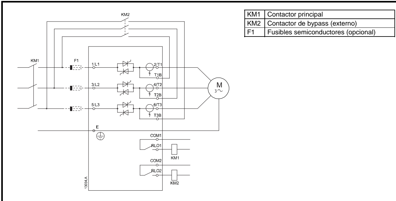
Figura 4-11 Conexiones de potencia - instalación directa (en línea), con bypass externo (D3-1x-0360-N a D3-16-1600-N)
