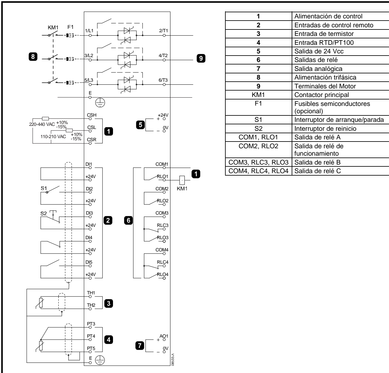
Figura 10-1 Instalación con interruptor principal
