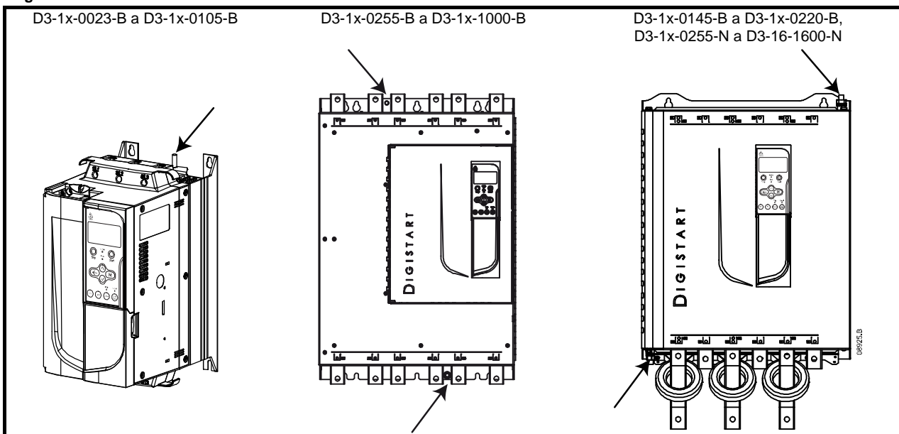
Figura 4-4 Localizaciones de los terminales de tierra
