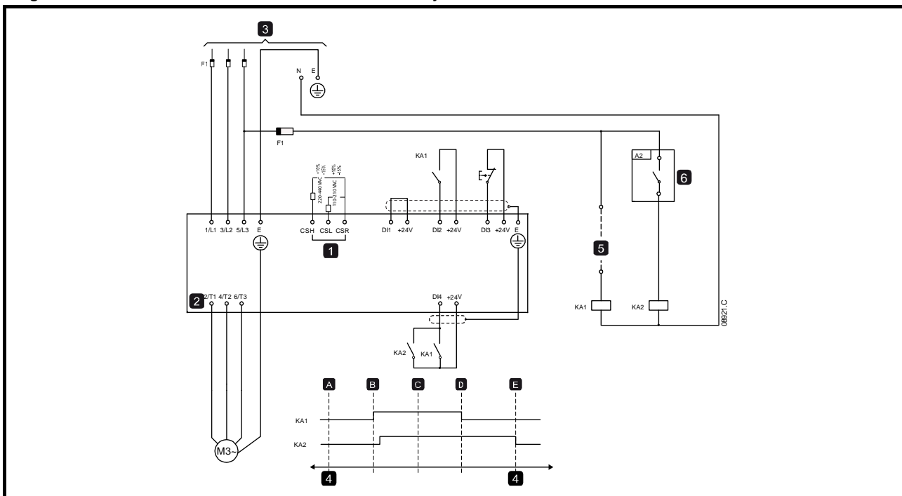
Figura 10-5 Freno DC con sensor externo de rotación del eje
