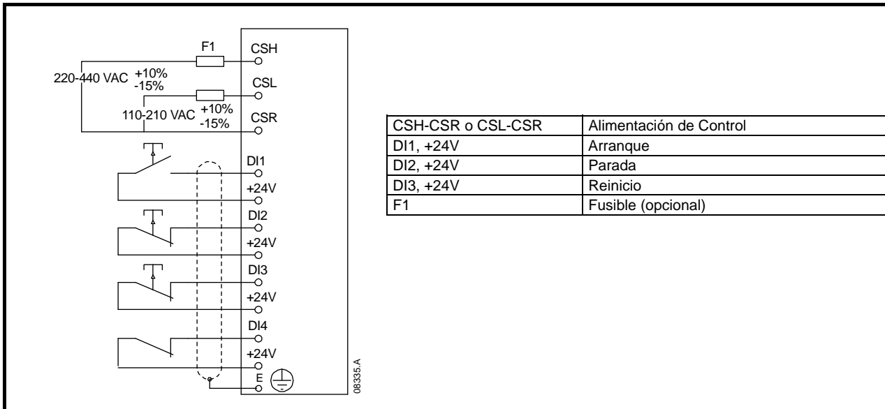
Figura 6-1 Terminales de control para una conexión básica
