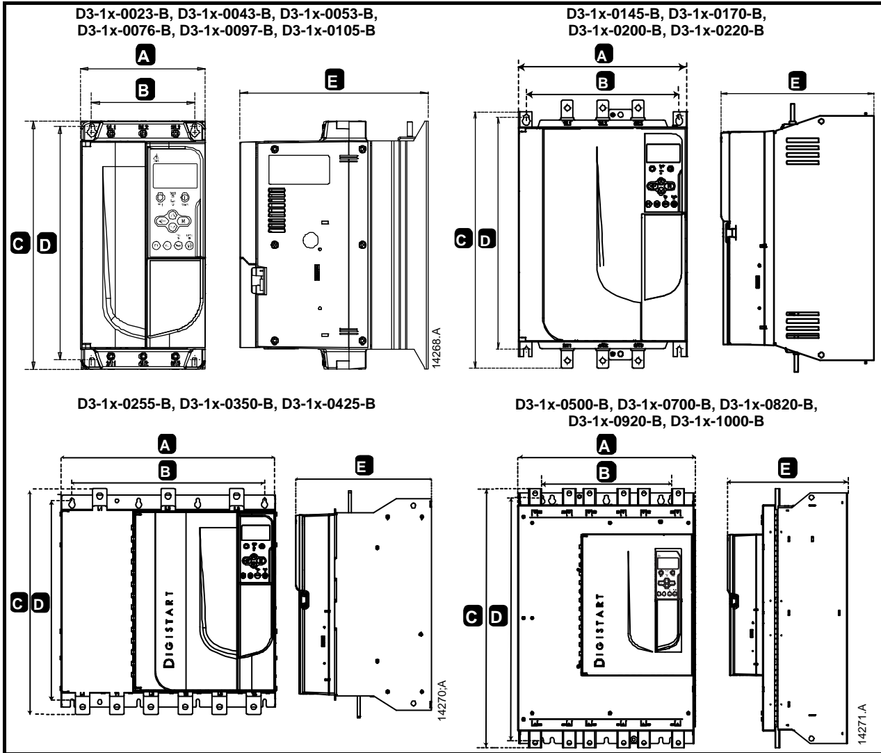
Figura 3-1 Dimensiones de la unidad (modelos con bypass)
