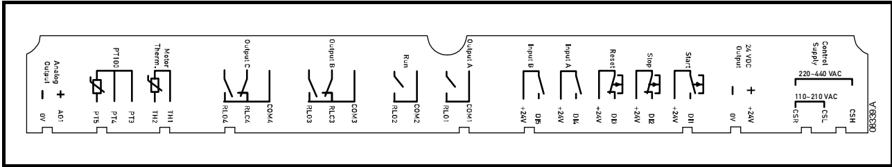
Figura 4-5 Disposición de terminales de control
