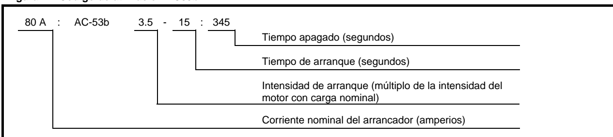
Figura 2-2 Código de utilización AC53b
