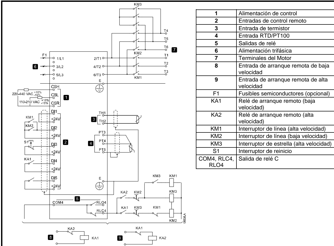
Figura 10-7 Motor de dos velocidades
