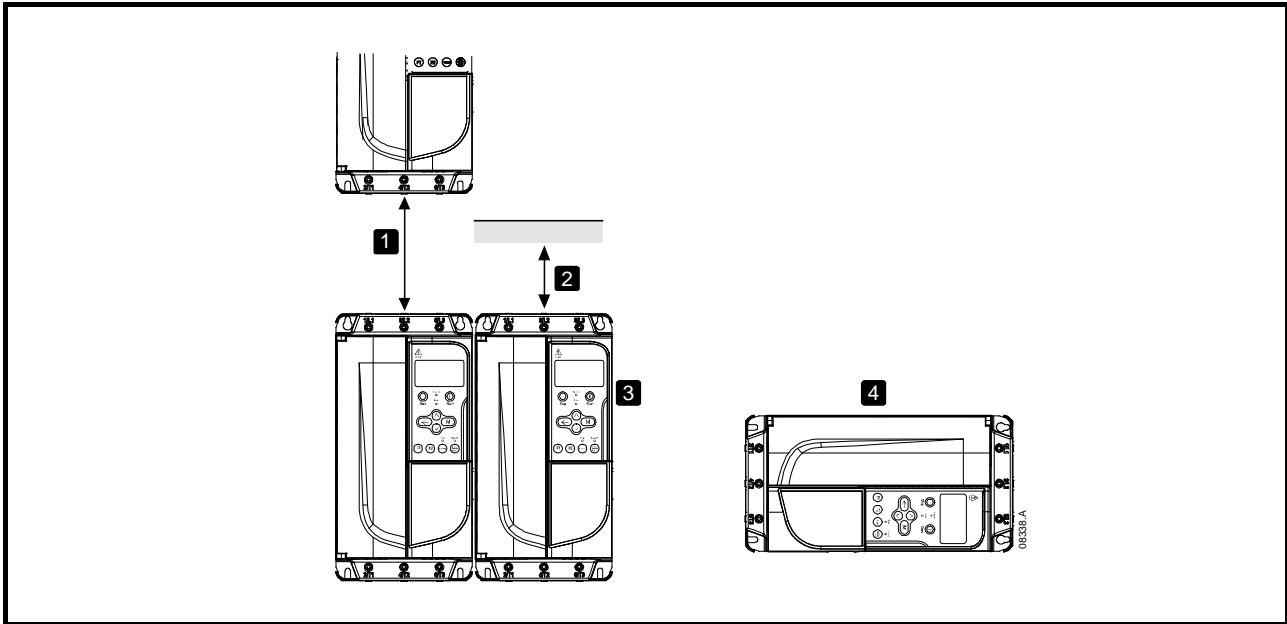
Figura 3-3 Tolerancias de montaje
