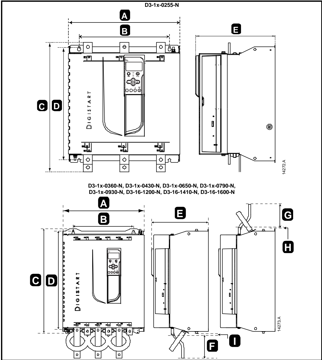
Figura 3-2 Dimensiones de la unidad (modelos sin bypass)
