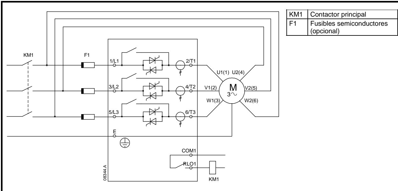
Figura 4-13 Conexiones de potencia - instalación en triángulo interno, con bypass interno
