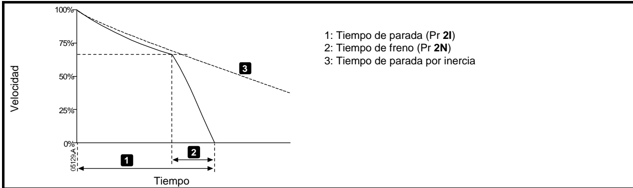
Figura 7-7 Parada con freno CC
