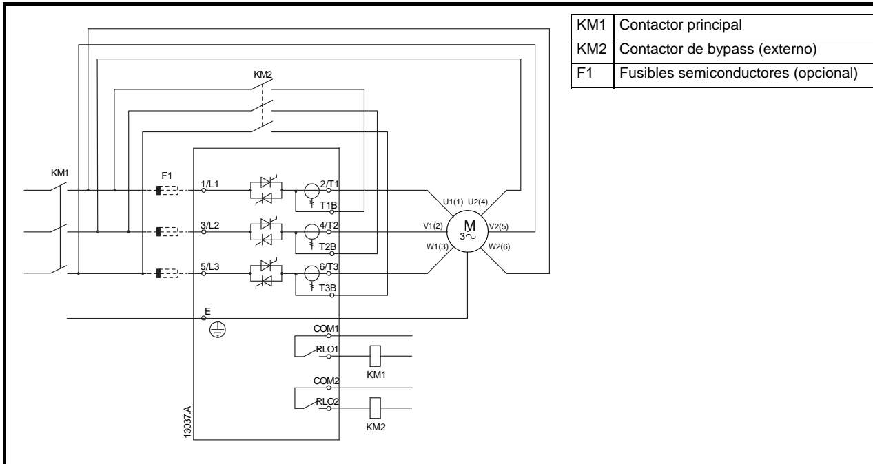
Figura 4-15 Conexiones de potencia - instalación en triángulo interno, con bypass externo (D3-1x-0360-N a D3-16-1600-N)
