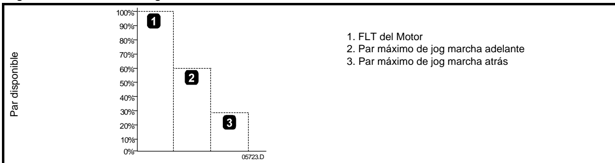
Figura 7-8 Funcionamiento Jog
