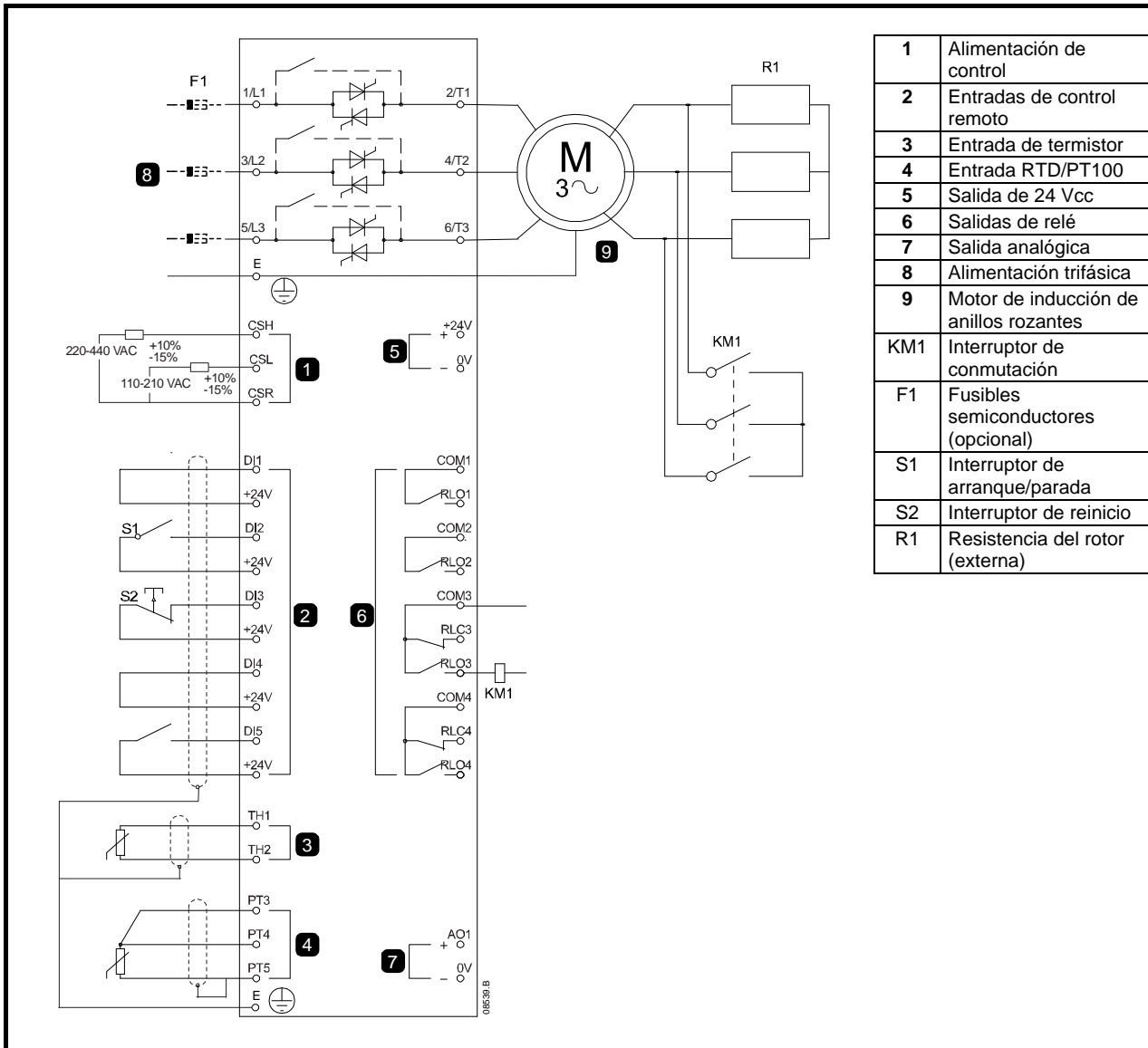
Figura 10-8 Motor de anillos rozantes
