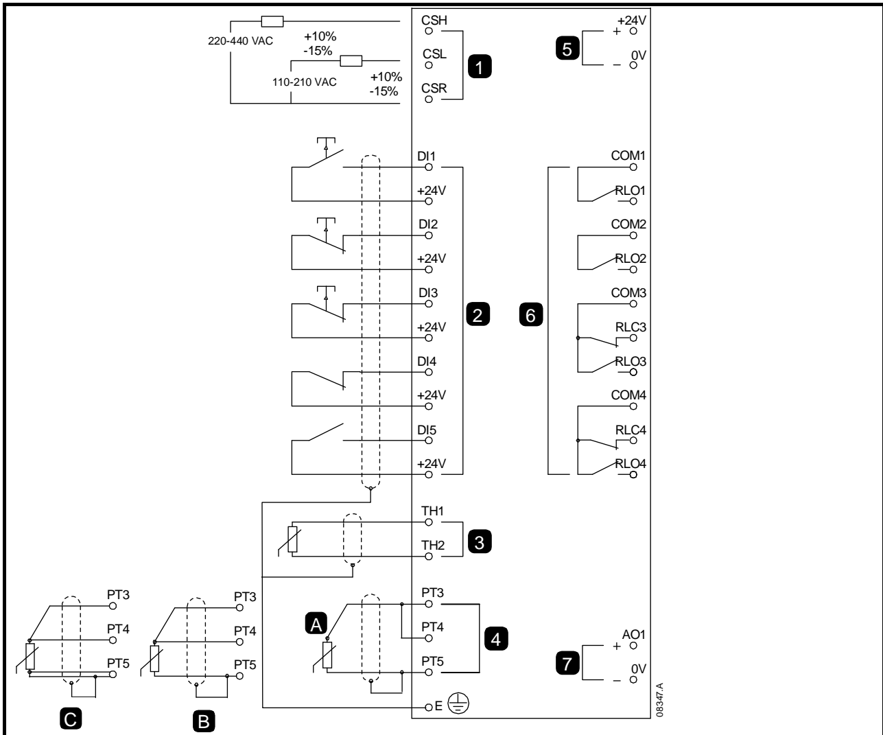
Figura 4-8 esquema eléctrico de Digistart D3
