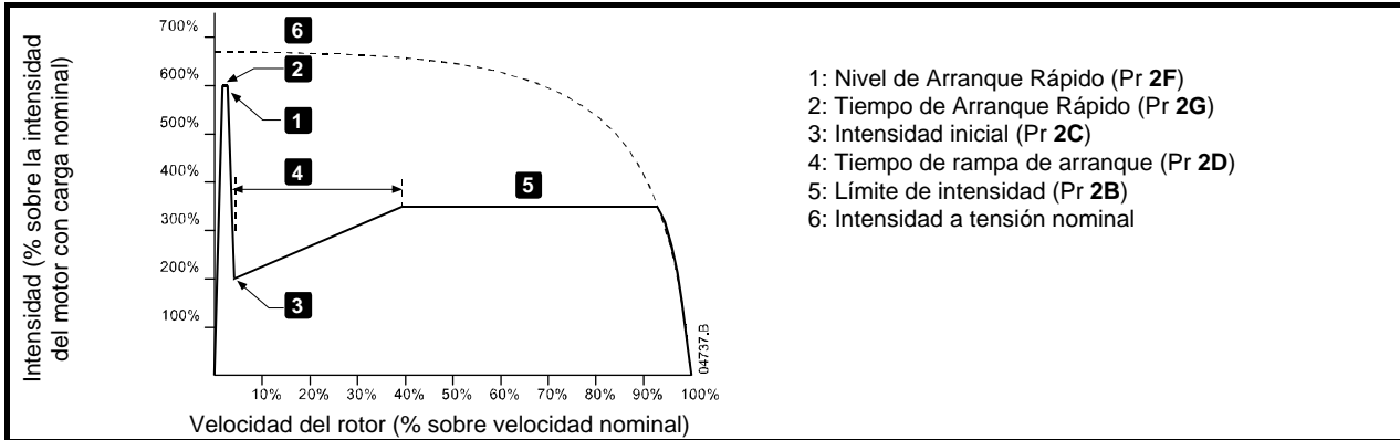
Figura 7-4 Arranque suave con rampa de intensidad con arranque rápido
