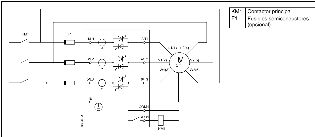
Figura 4-16 Conexiones de potencia - instalación en triángulo interno, sin bypass
