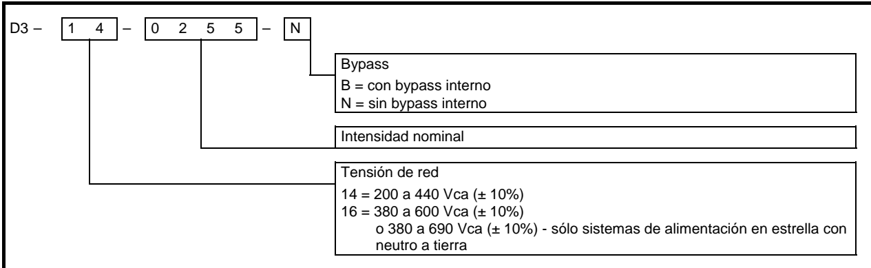
Figura 2-1 Explicación del código de modelo
