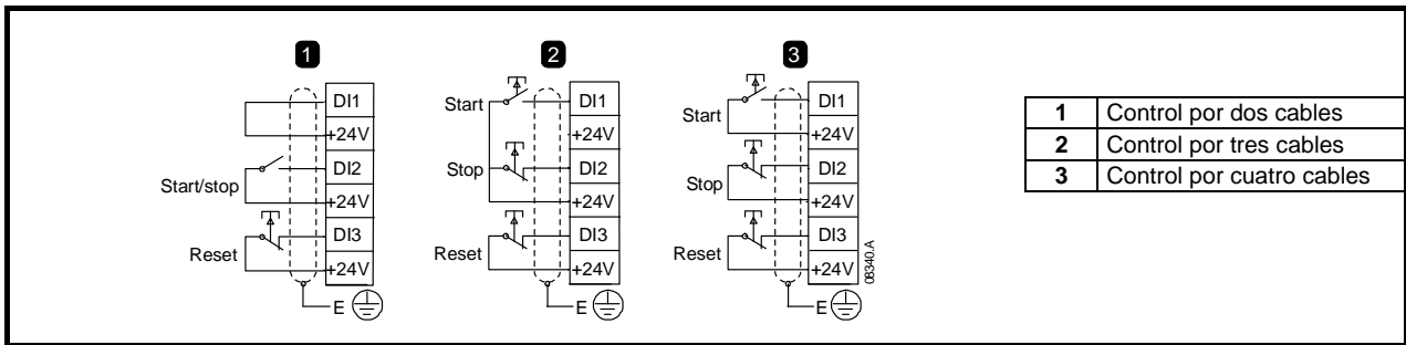
Figura 4-6 Opciones del cableado de control
