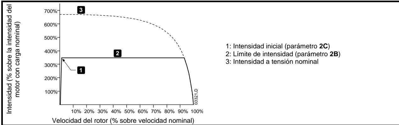
Figura 7-1 Arranque suave con intensidad constante
