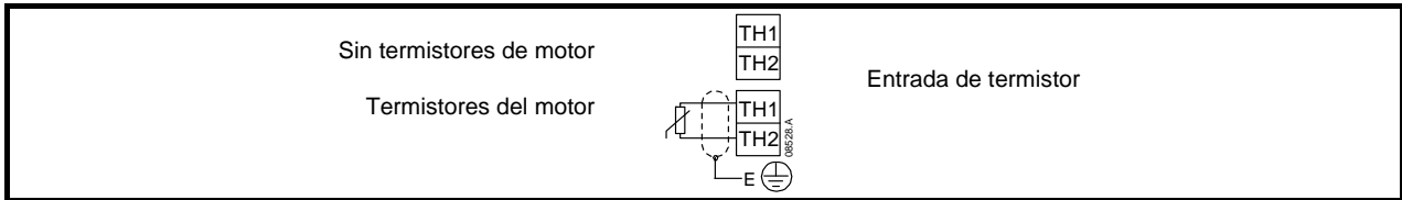
Figura 4-7 Conexión del termistor del motor
