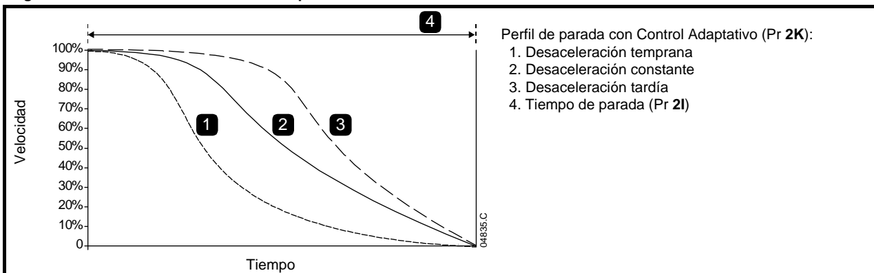
Figura 7-6 Parada suave con Control Adaptativo
