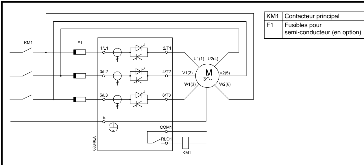
Figure 4-16 Connexions de puissance - connexion 6 fils, sans bypass
