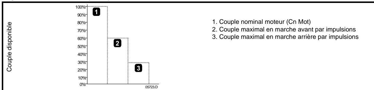
Figure 7-8 Mode de marche par impulsions
