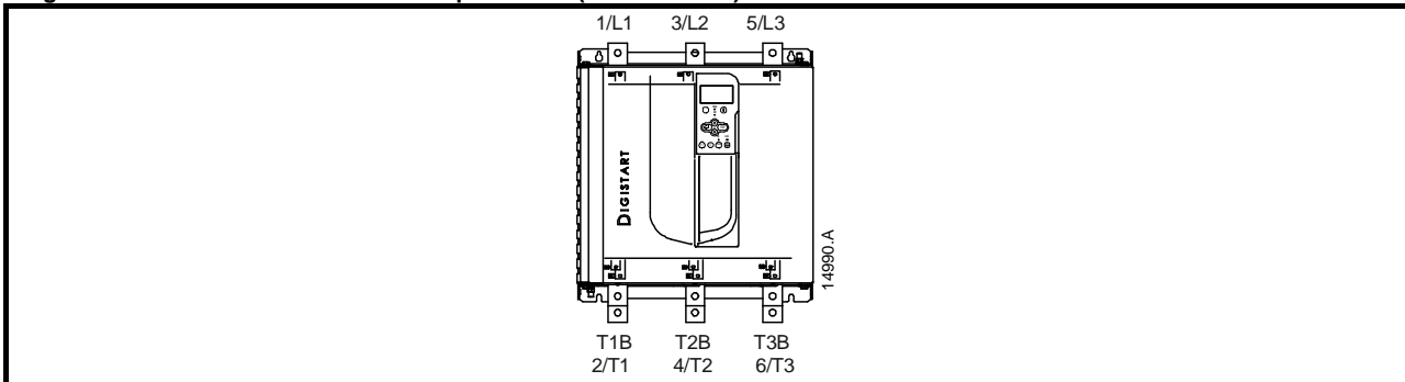
Figure 4-2 Bornes d'entrée et sortie de puissance (D3-1x-0255-N)
