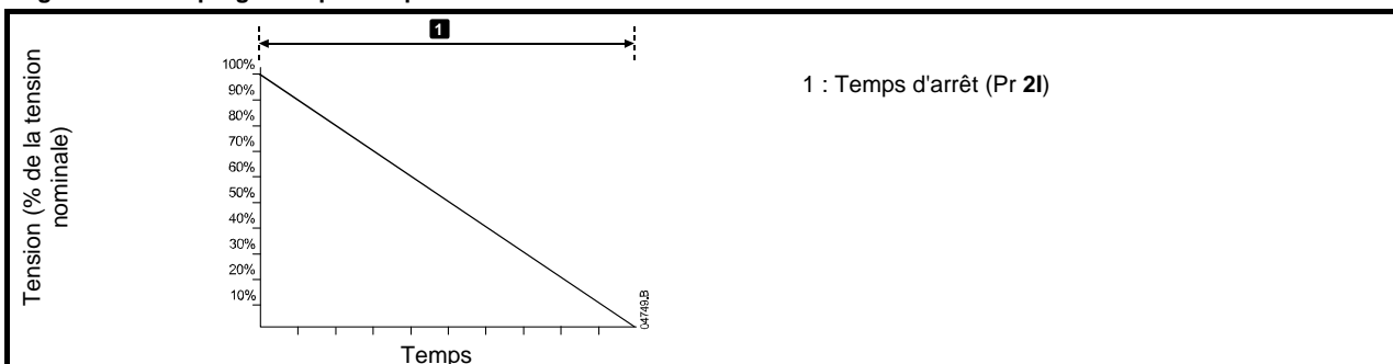
Figure 7-5 Arrêt progressif par rampe de tension
