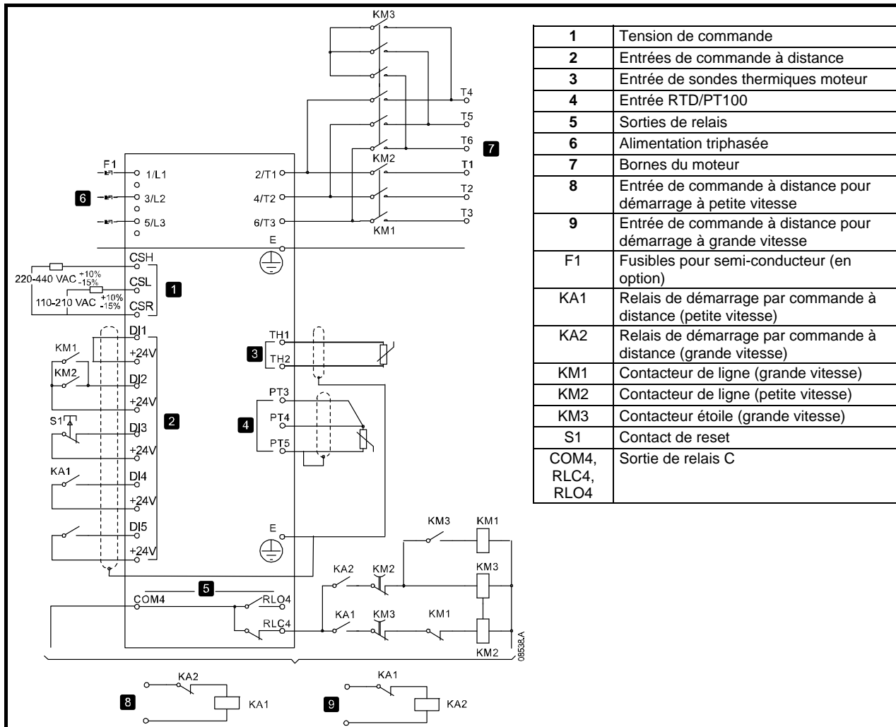
Figure 10-7 Moteur à deux vitesses
