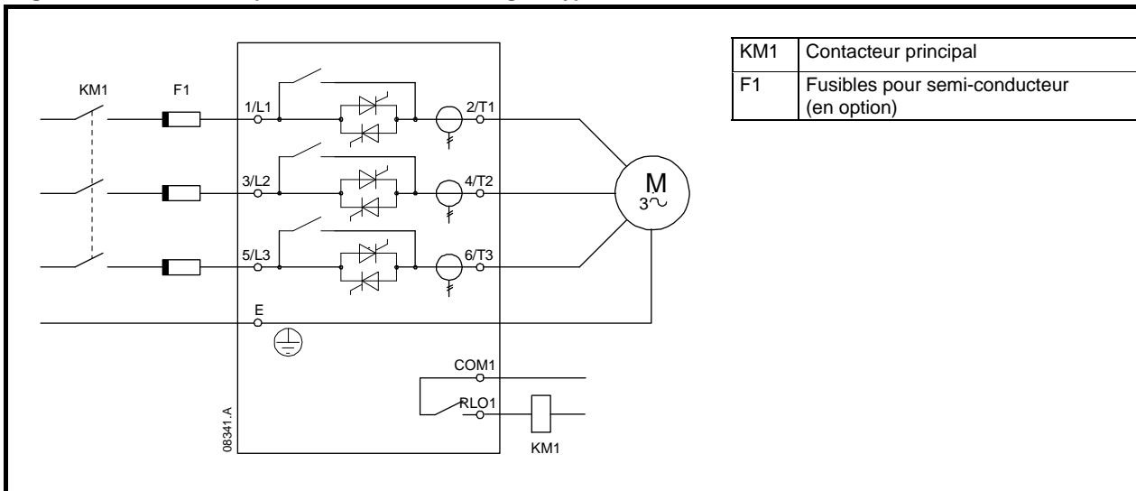
Figure 4-9 Connexions de puissance - connexion en ligne, bypass interne
