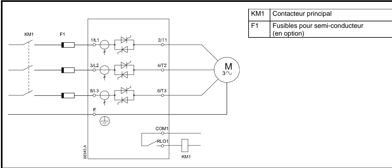
Figure 4-12 Connexions de puissance - connexion en ligne, sans bypass
