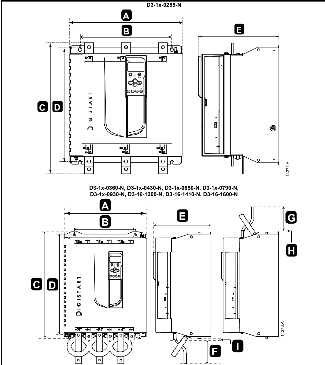
Figure 3-2 Dimensions des appareils (modèles sans circuit bypass)
