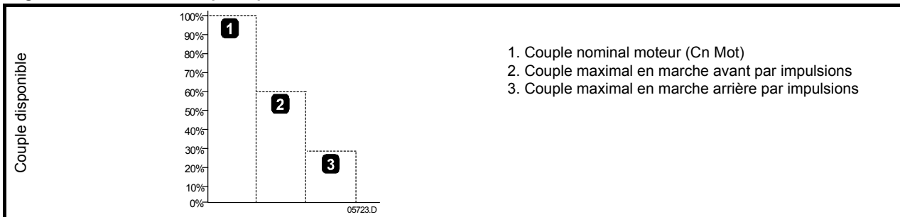
Figure 7-8 Mode de marche par impulsions
