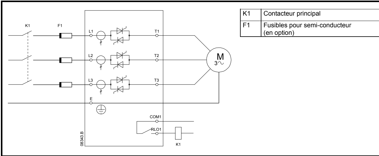
Figure 4-12 Connexions de puissance - connexion en ligne, sans bypass
