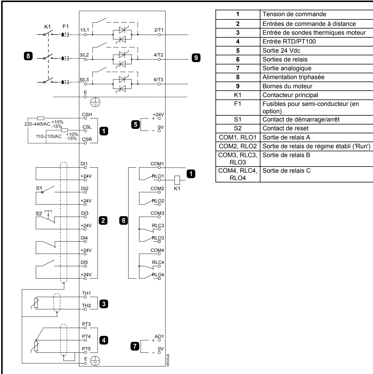
Figure 10-1 Installation avec un contacteur principal
