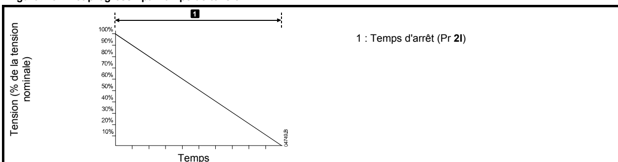
Figure 7-5 Arrêt progressif par rampe de tension
