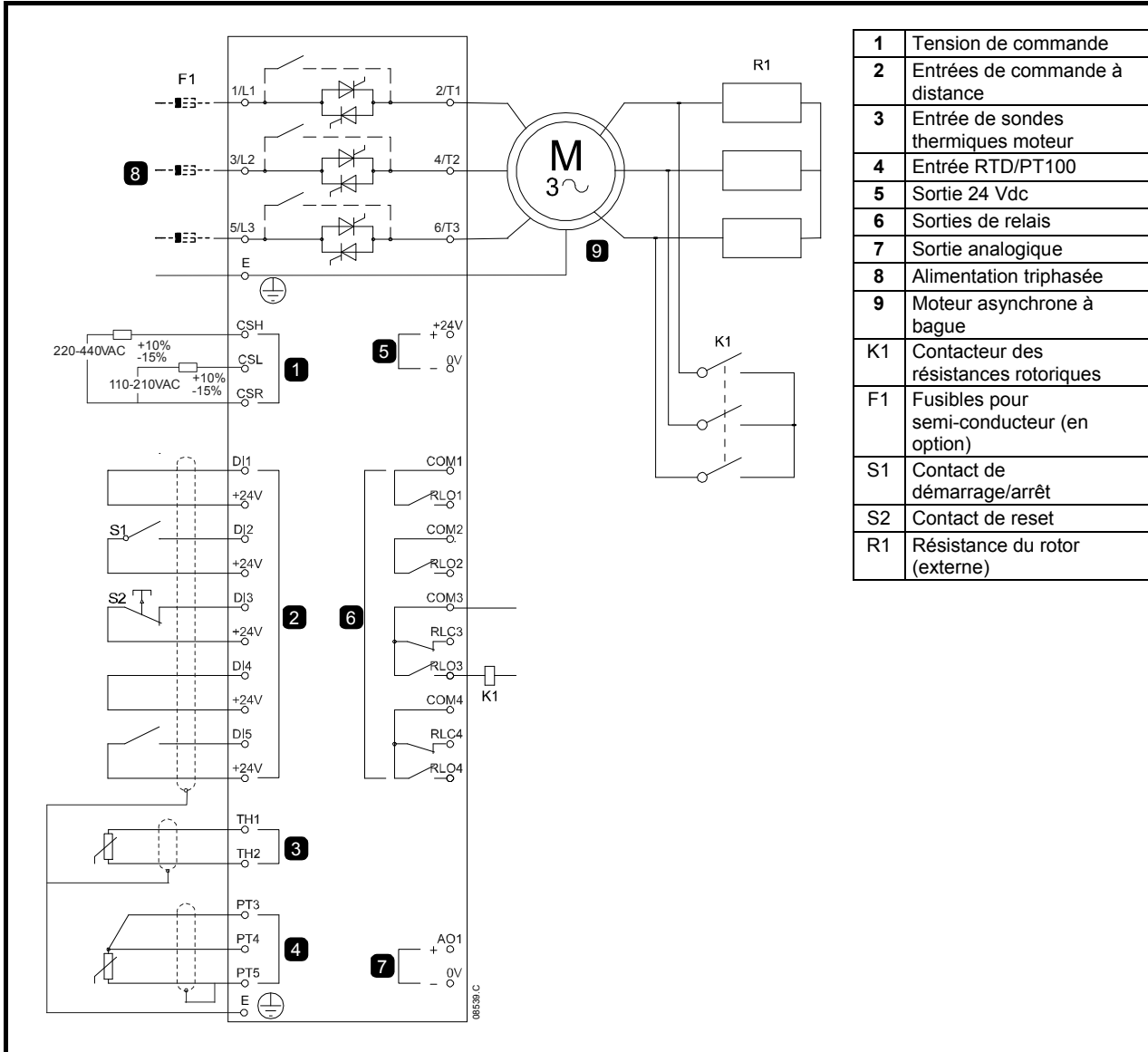
Figure 10-8 Moteur à bague
