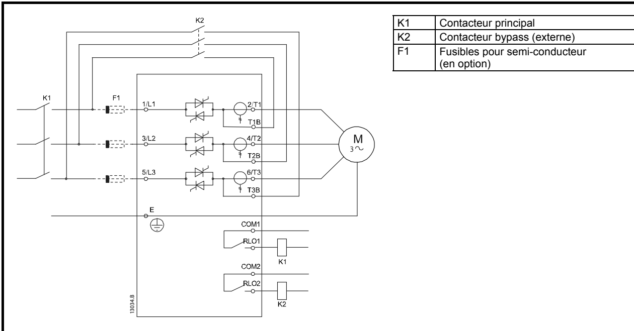
Figure 4-11 Connexions de puissance - connexion en ligne, bypass externe (D3-1x-0360-N à D3-16-1600-N)
