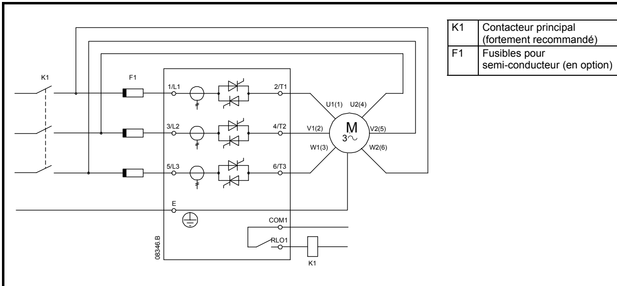
Figure 4-16 Connexions de puissance - connexion 6 fils, sans bypass
