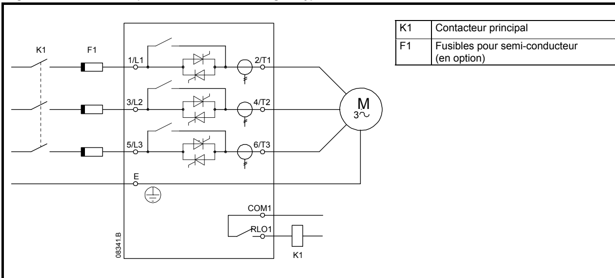
Figure 4-9 Connexions de puissance - connexion en ligne, bypass interne
