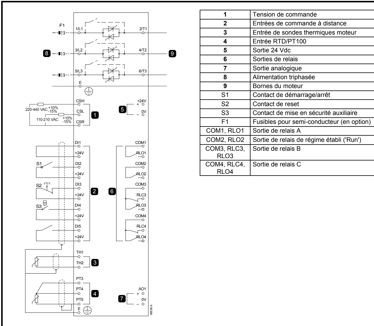
Figure 10-4 Circuit de mise en sécurité auxiliaire
