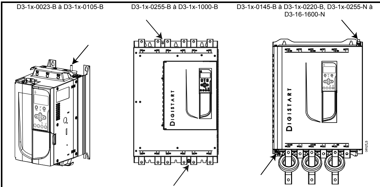
Figure 4-4 Localisation des bornes de terre
