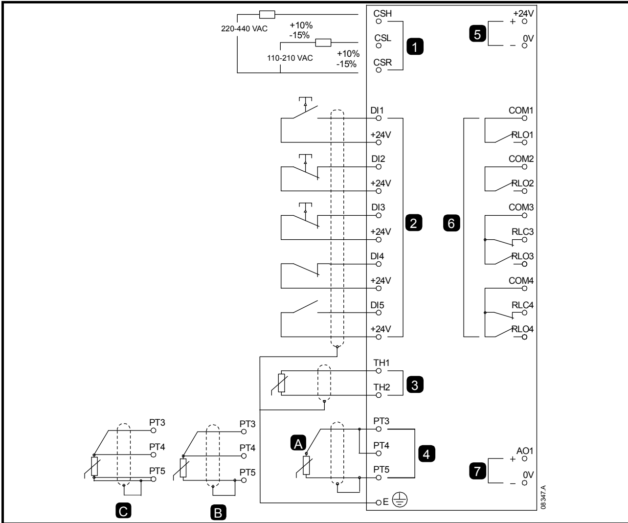
Figure 4-8 Schéma électrique du Digistart D3
