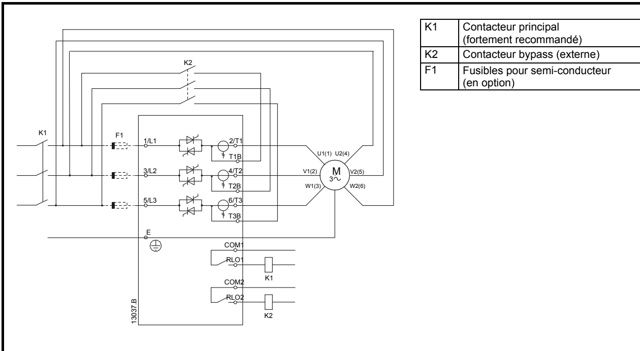
Figure 4-15 Connexions de puissance - connexion 6 fils, bypass externe (D3-1x-0360-N à D3-16-1600-N)
