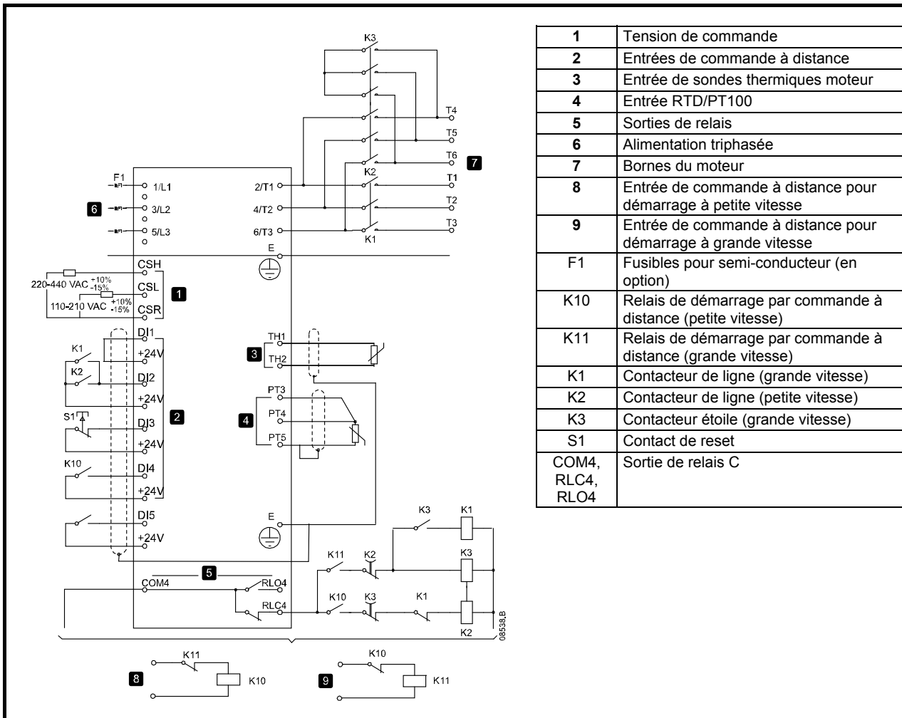
Figure 10-7 Moteur à deux vitesses
