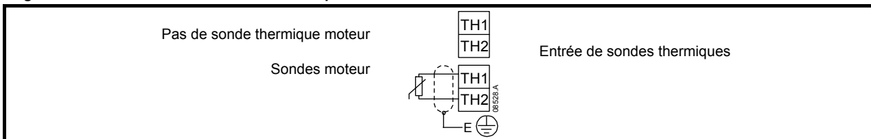
Figure 4-7 Raccordement des sondes thermiques moteur
