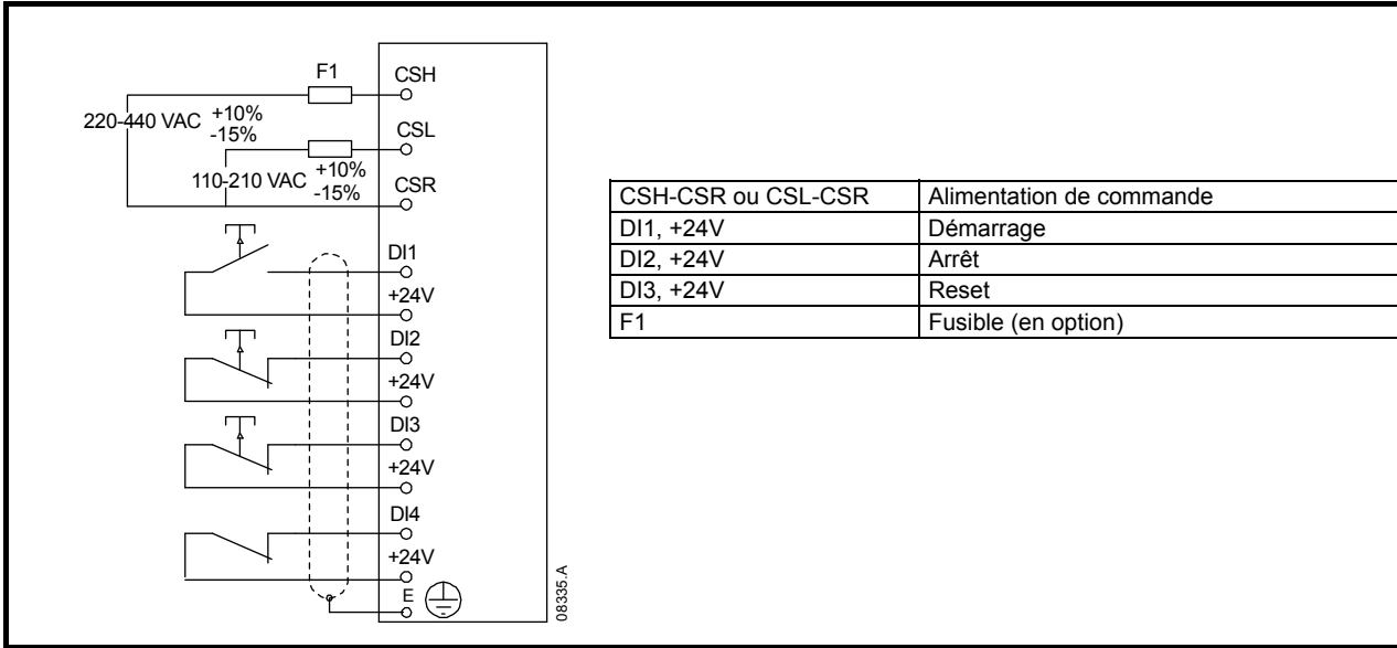
Figure 6-1 Bornes de commande pour connexion de base
