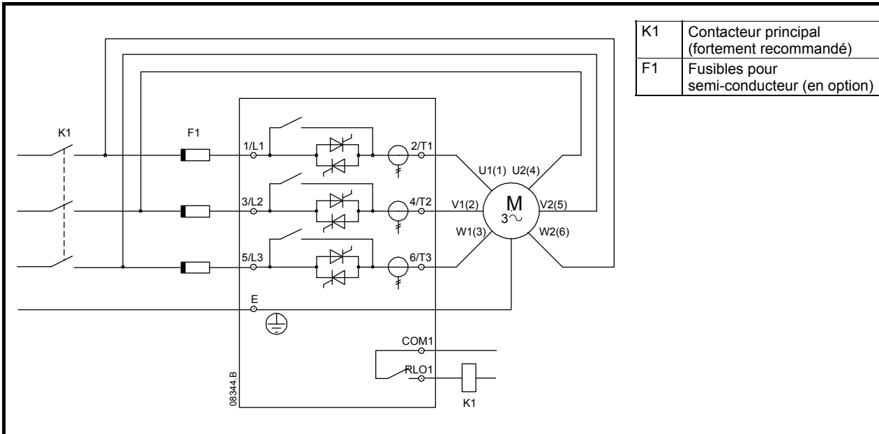
Figure 4-13 Connexions de puissance - connexion 6 fils, bypass interne
