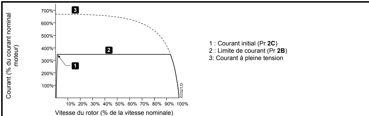
Figure 7-1 Démarrage progressif par courant constant
