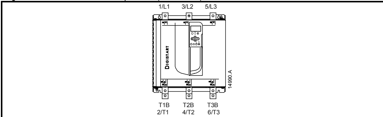
Figure 4-2 Bornes d'entrée et sortie de puissance (D3-1x-0255-N)
