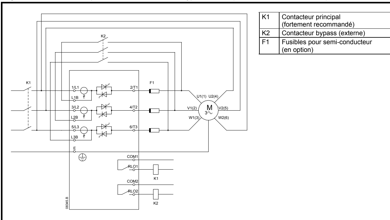
Figure 4-15 Connexions de puissance - connexion 6 fils, bypass externe (D3-1x-0360-N à D3-16-1600-N)
