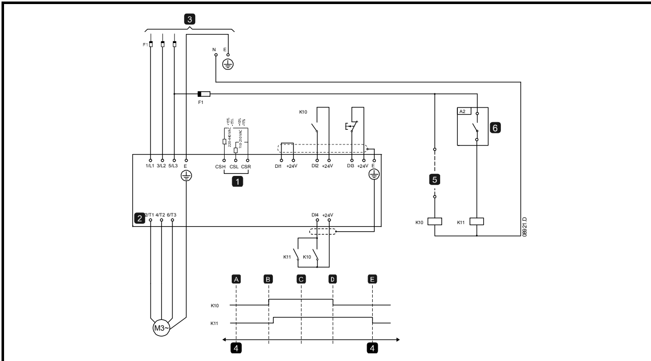
Figure 10-5 Freinage DC avec capteur de vitesse nulle externe
