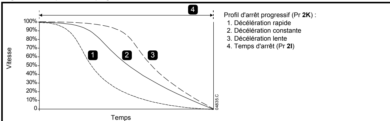
Figure 7-6 Arrêt par contrôle progressif
