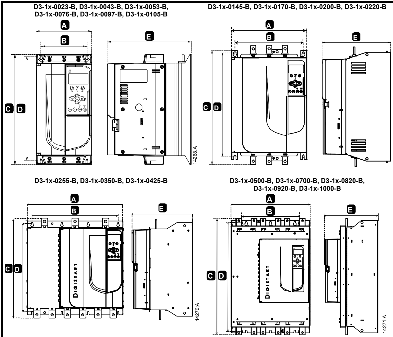
Figure 3-1 Dimensions des appareils (modèles à circuit bypass)
