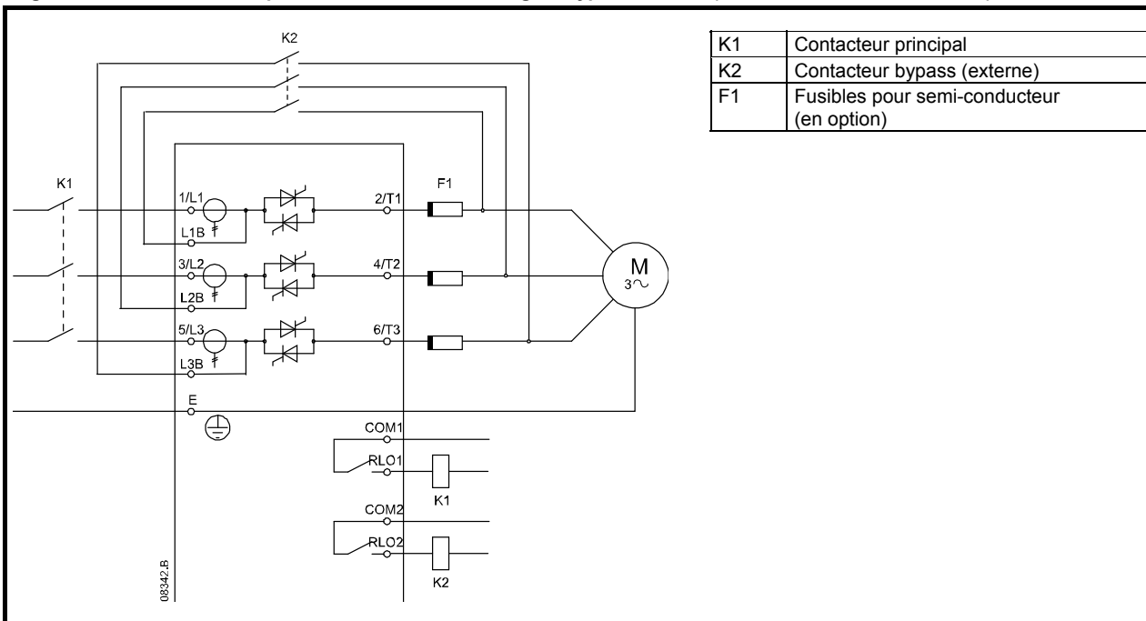
Figure 4-11 Connexions de puissance - connexion en ligne, bypass externe (D3-1x-0360-N à D3-16-1600-N)
