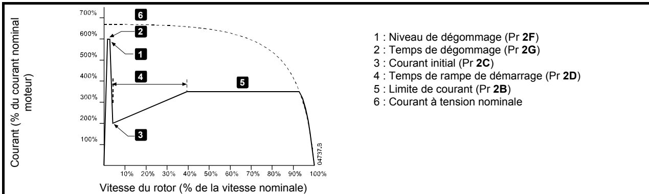
Figure 7-4 Démarrage par rampe de courant avec dégommeage
