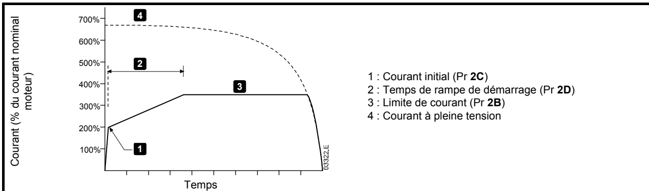
Figure 7-2 Démarrage progressif par rampe de courant
