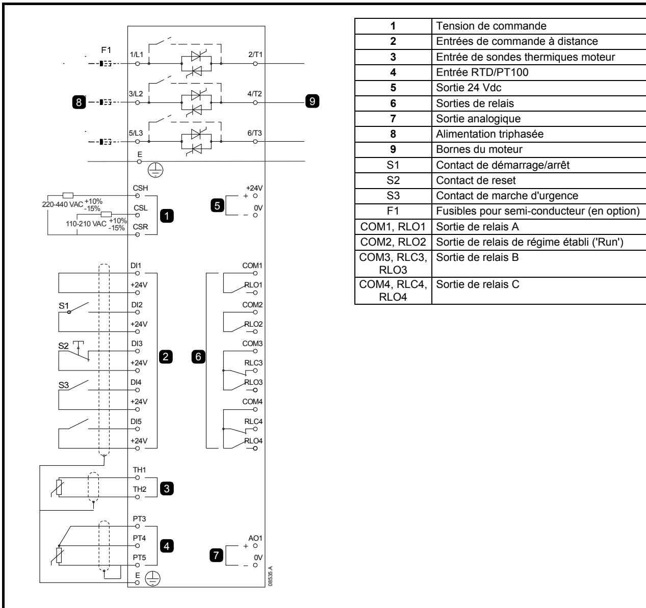
Figure 10-3 Opération en marche d'urgence
