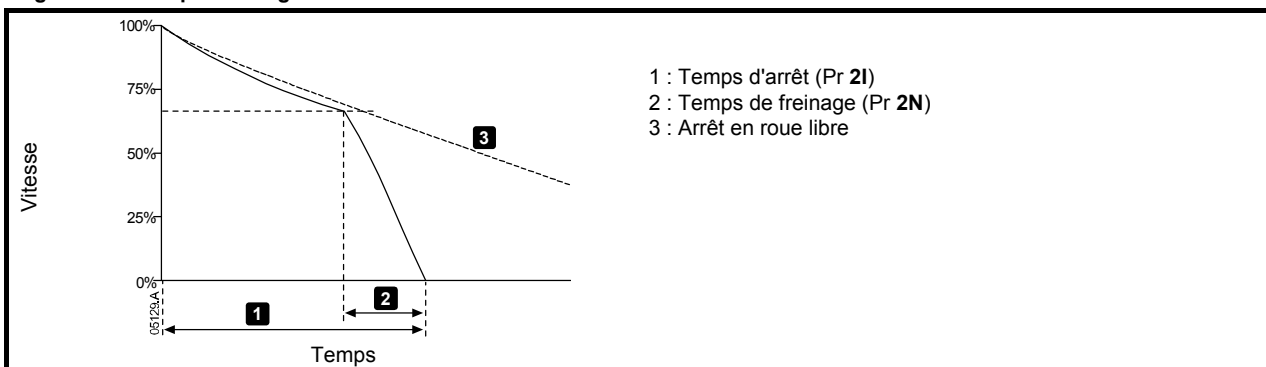
Figure 7-7 Arrêt par freinage DC
