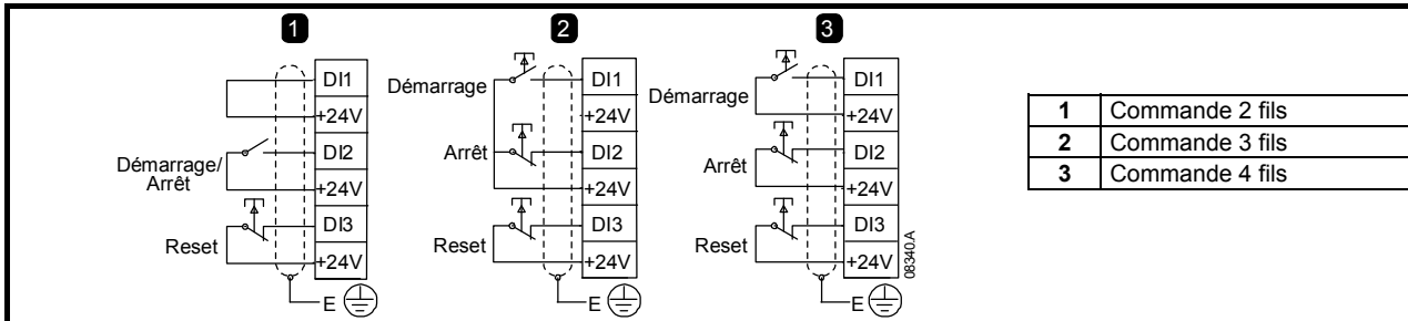
Figure 4-6 Options de câblage de commande
