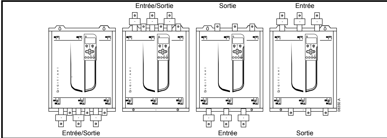
Figure 3-4 Options de configuration des barres de puissance (D3-1x-0360-N à D3-16-1600-N)
