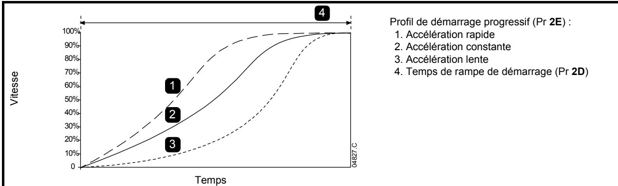
Figure 7-3 Démarrage par contrôle progressif
