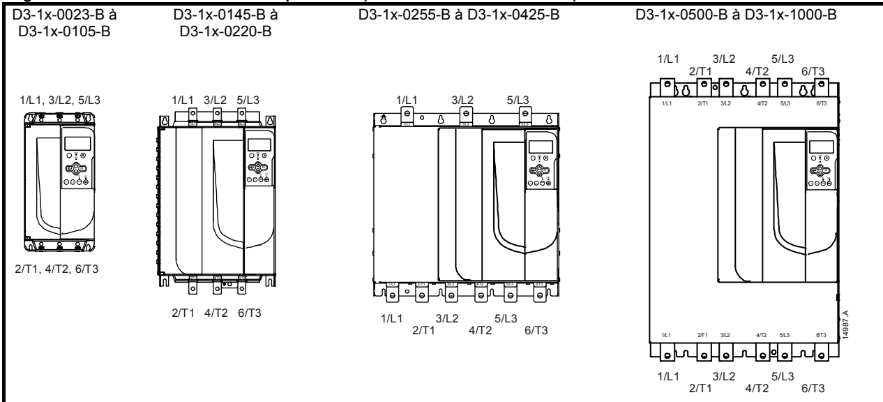
Figure 4-1 Bornes d'entrée et sortie de puissance (D3-1x-0023-B à D3-1x-1000-B)
