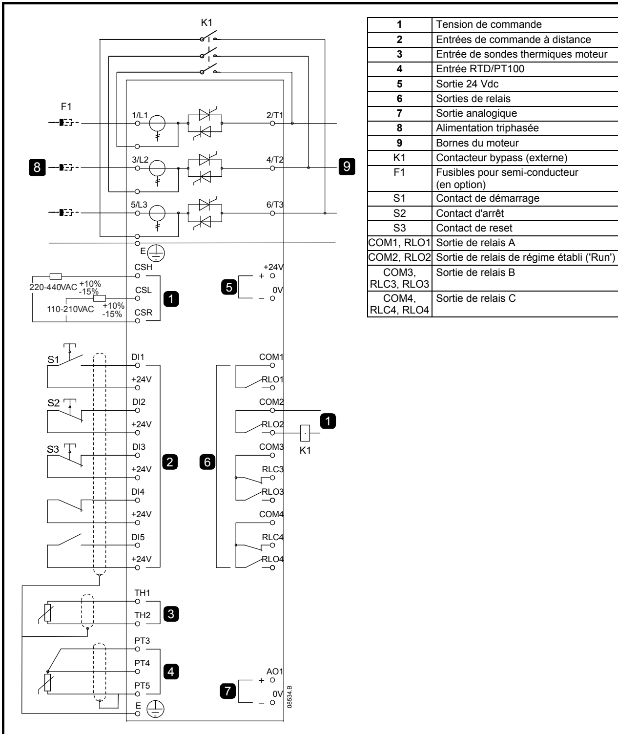
Figure 10-2 Installation avec un contacteur bypass
