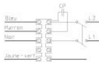
Schéma de branchement du coffret
