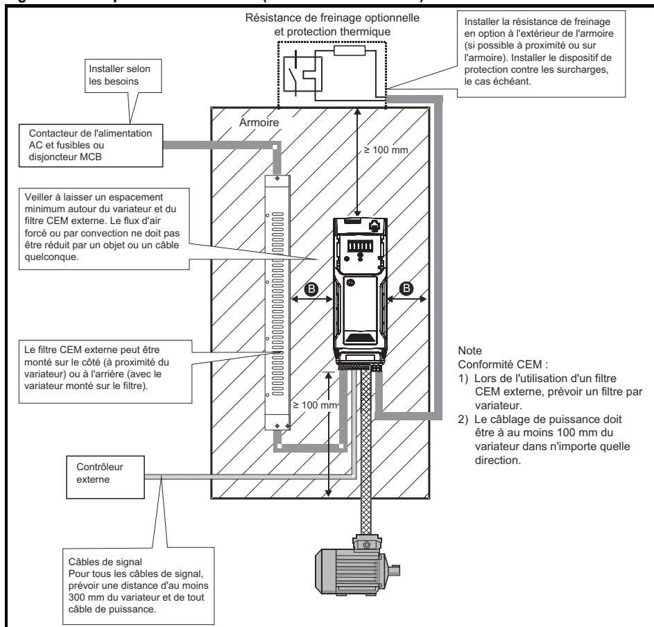
Figure 3-7 Disposition de l'armoire (Unidrive M400 illustré)
