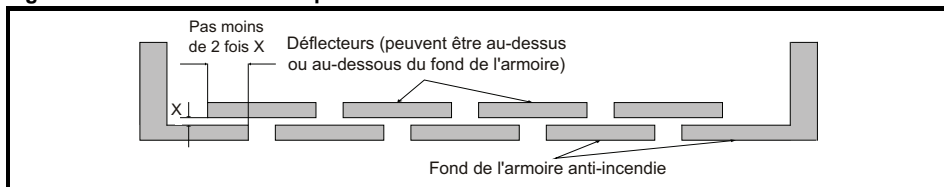
Figure 3-2 Présentation d'un pare-flammes sur une armoire anti-incendie
