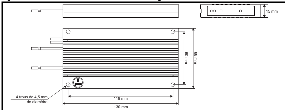
Figure 3-20 Dimensions de la résistance de freinage
