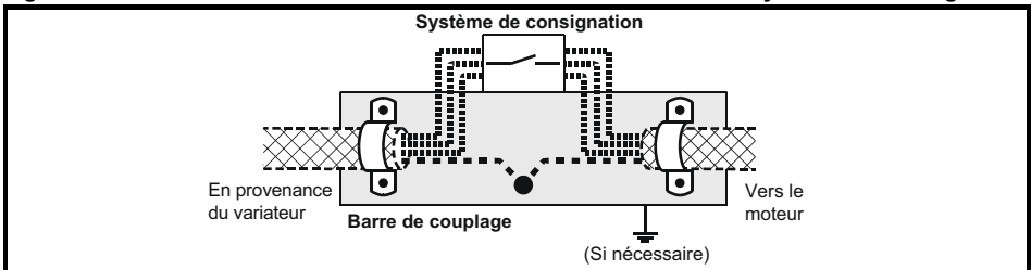
Figure 4-23 Raccordement du câble moteur à un contacteur ou un système de consignation
