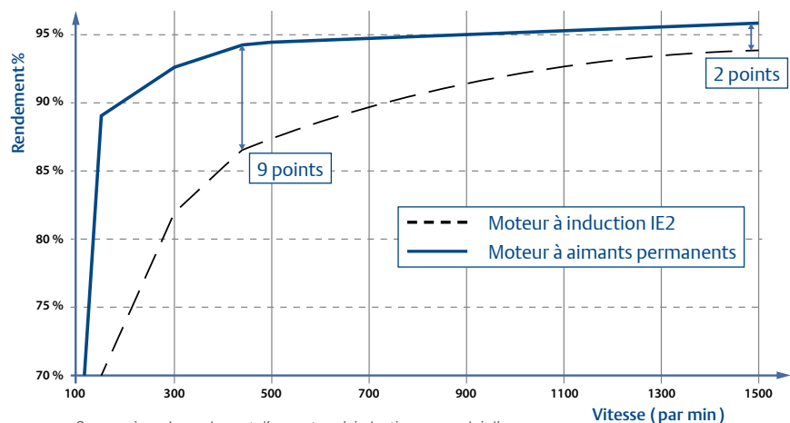
Comparaison du rendement d'un moteur à induction avec celui d'un moteur à aimants permanents à différents régimes (moteur de 55KW)
