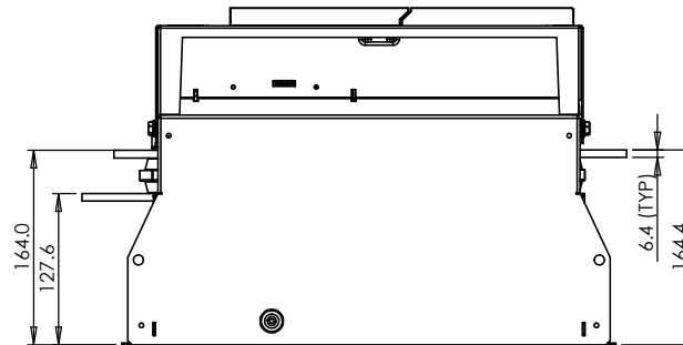
RIGHT ELEVATION
