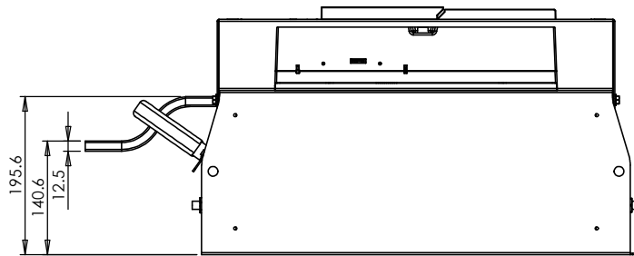
RIGHT ELEVATION
